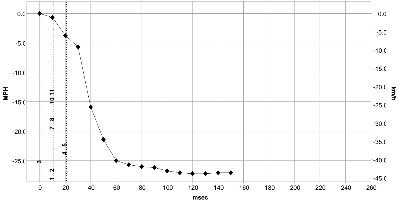
Longitudinal Delta-V
