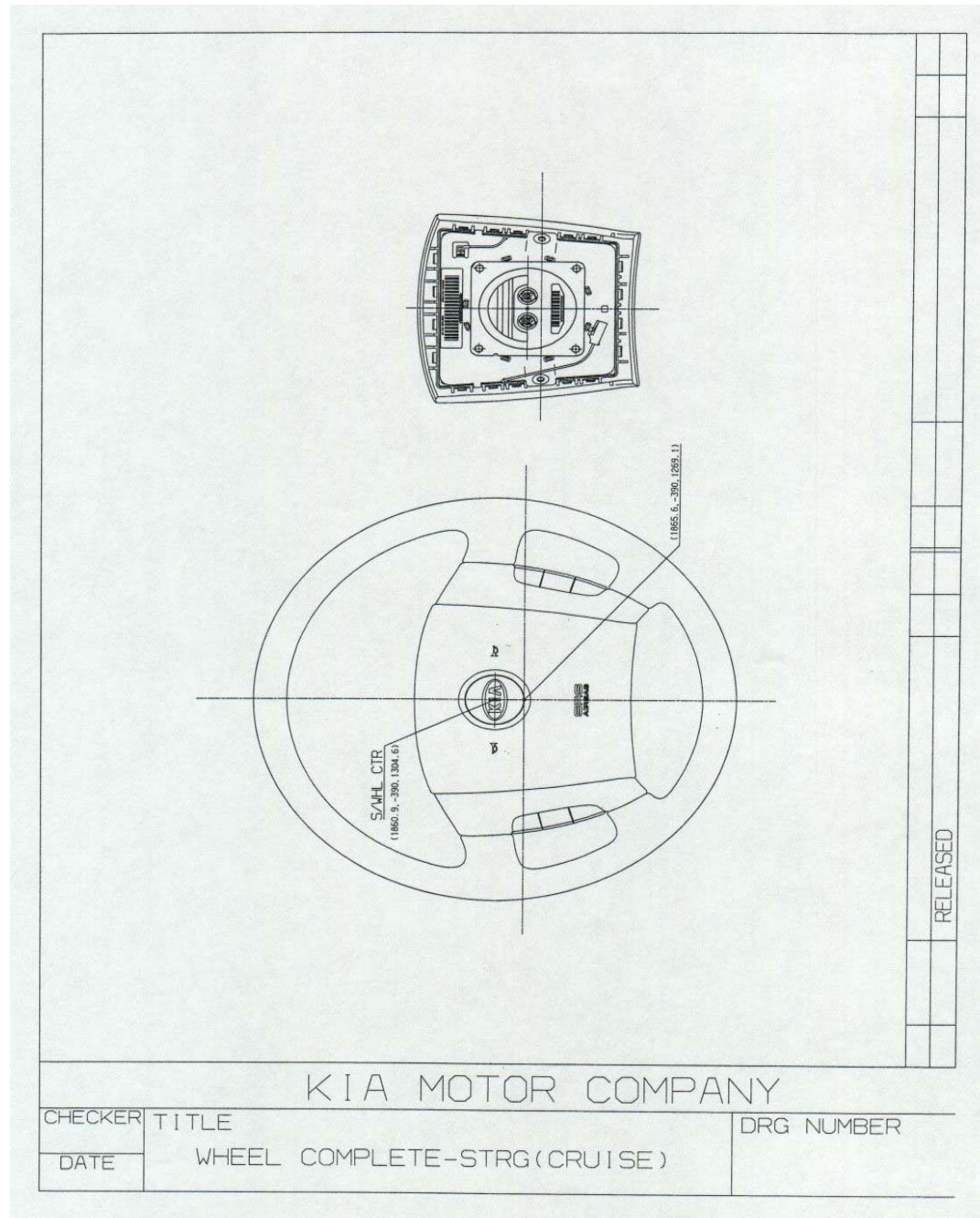
Driver Airbag Geometric Center (2005 Kia Sorento)
