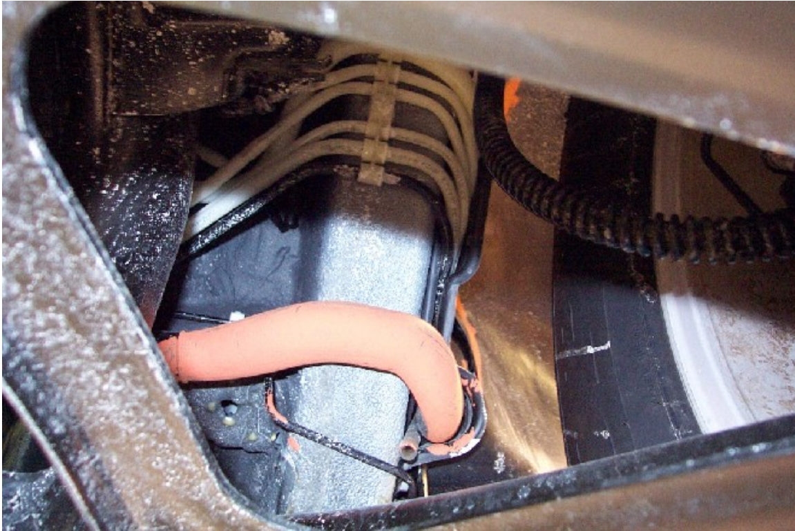
33. Tuyau de remplissage et vapeur. Filler and vapor pipe.
