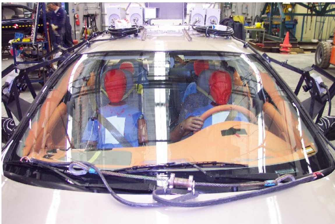
29. Pare-brise, avant essai. Windshield, pre-test.
