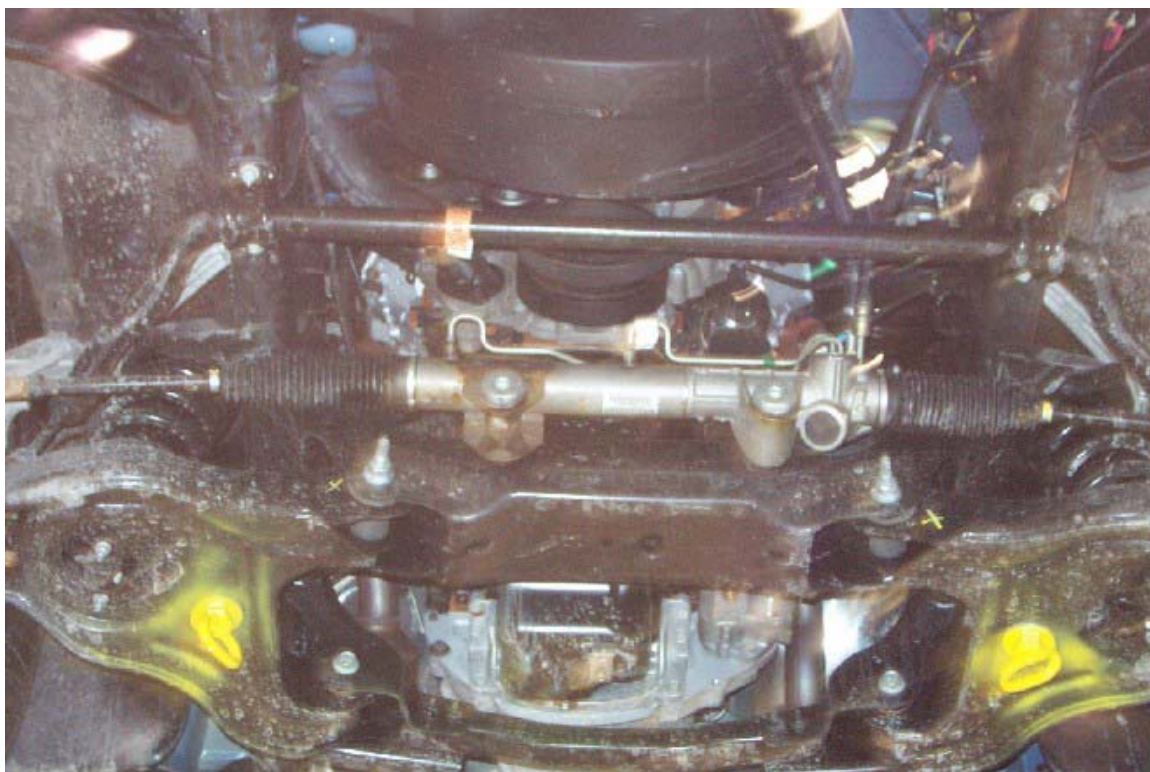
37. Vue du dessous du compartiment moteur, avant essai. Under view of the engine compartment , pre-test.
