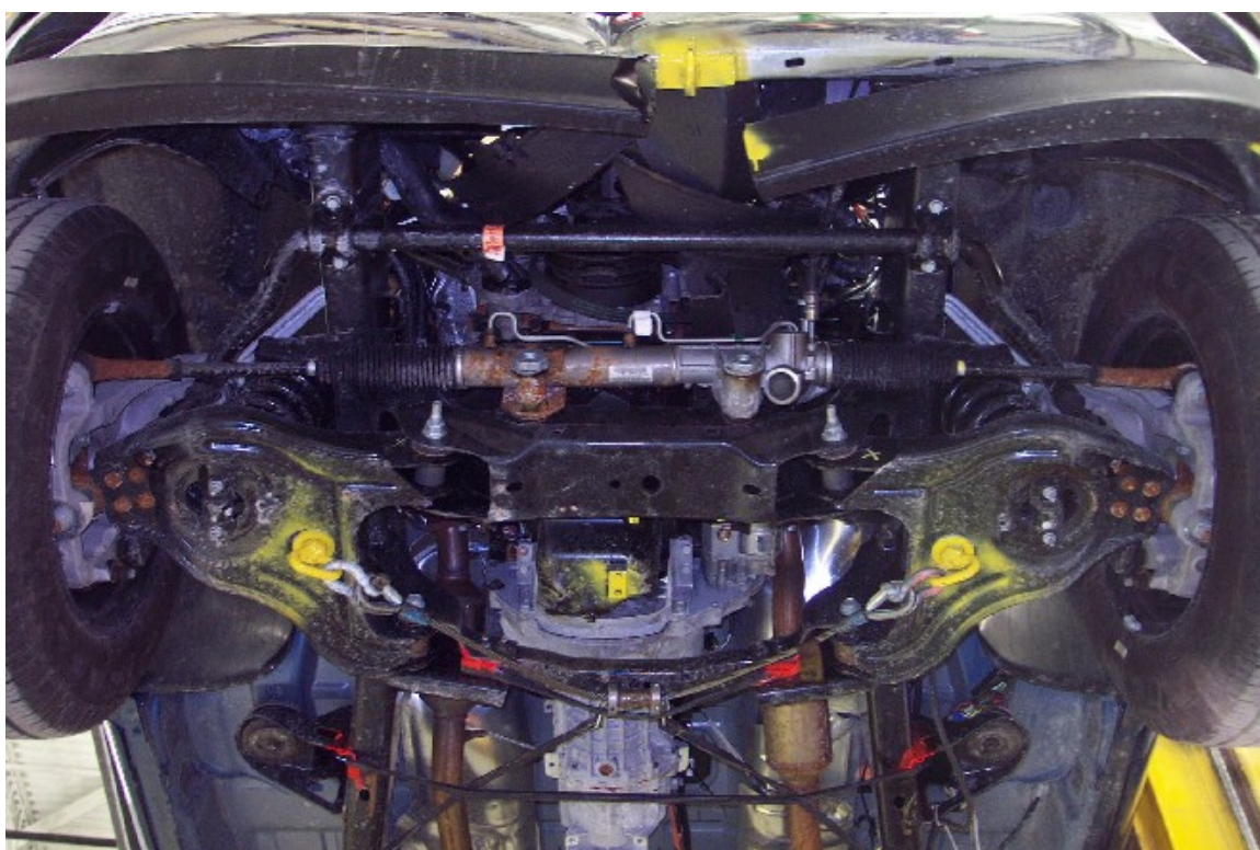
38. Vue du dessous du compartiment moteur, après essai. Under view of the engine compartment , post-test.
