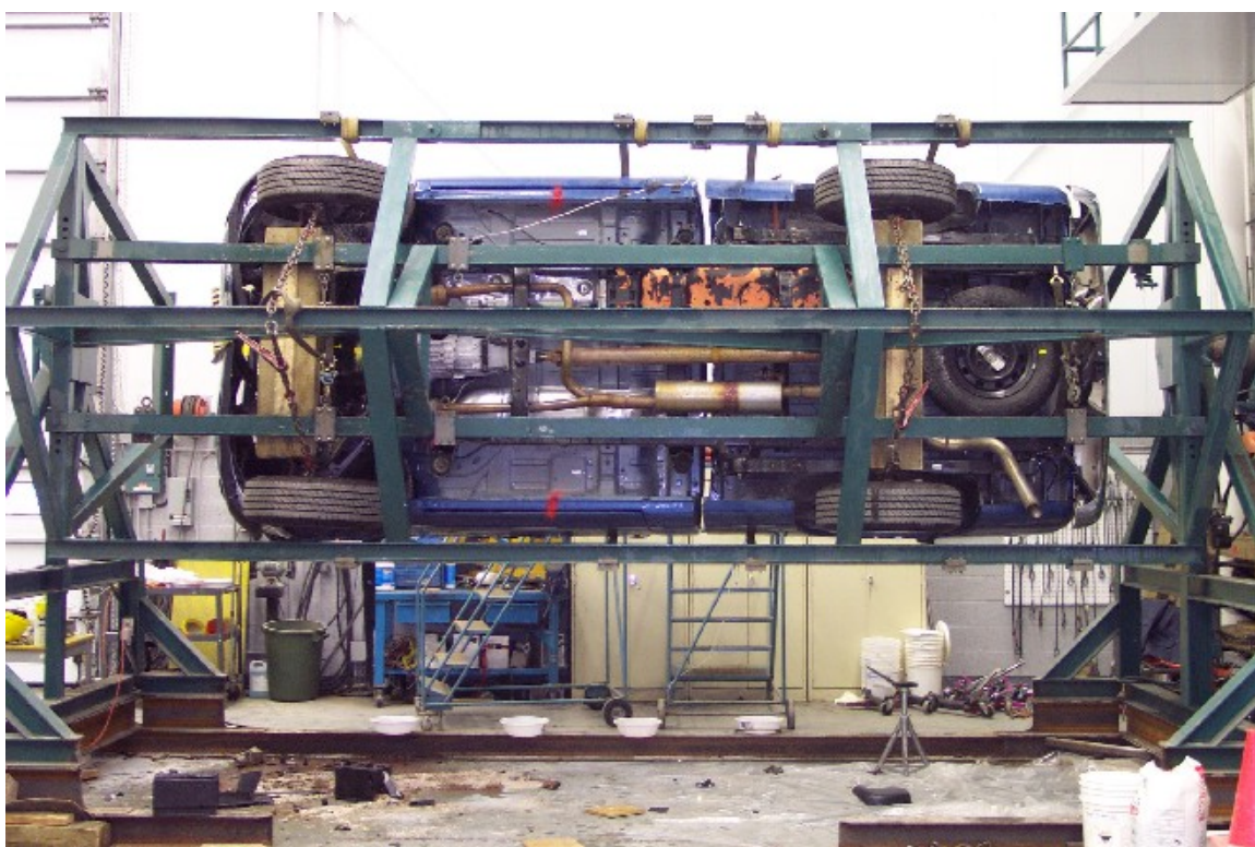
42. Vue du véhicule sur culbuteur à 270°. View of the vehicle on the roll over device at 270°.
