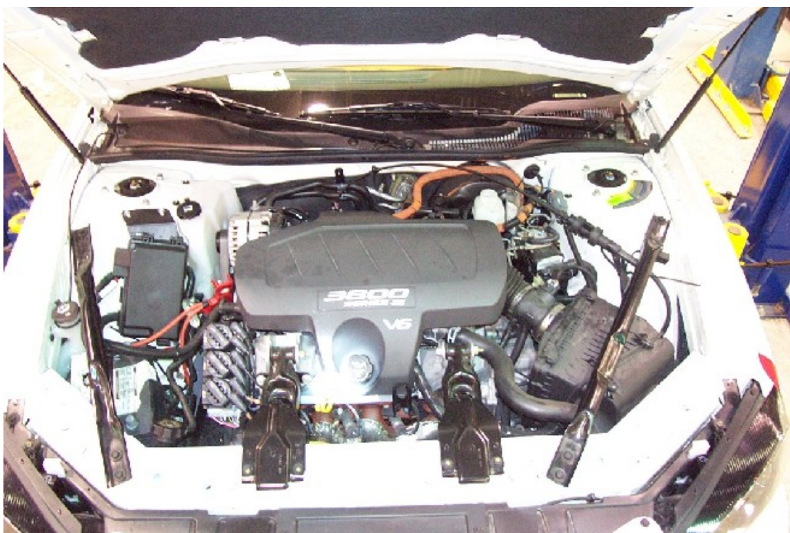
39. Vue du compartiment moteur du véhicule d'essai, avant essai. Engine compartment view of the vehicle, pre-test.
