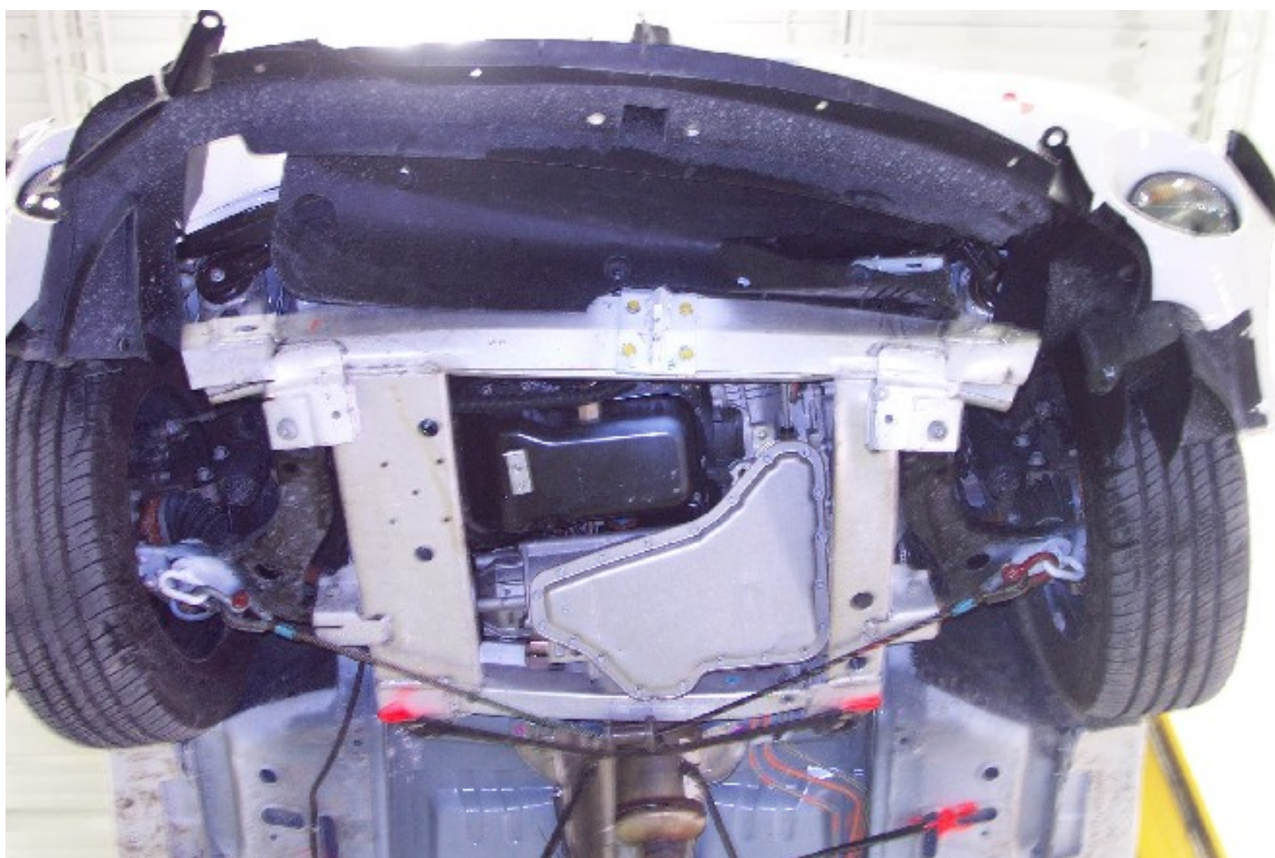
42. Vue du dessous du compartiment moteur, après essai. Under view of the engine compartment , post-test.
