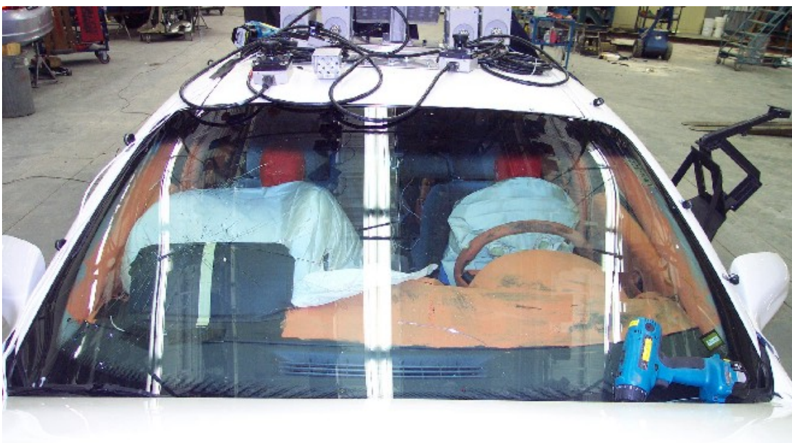
29. Pare-brise, avant essai. Windshield, pre-test.
