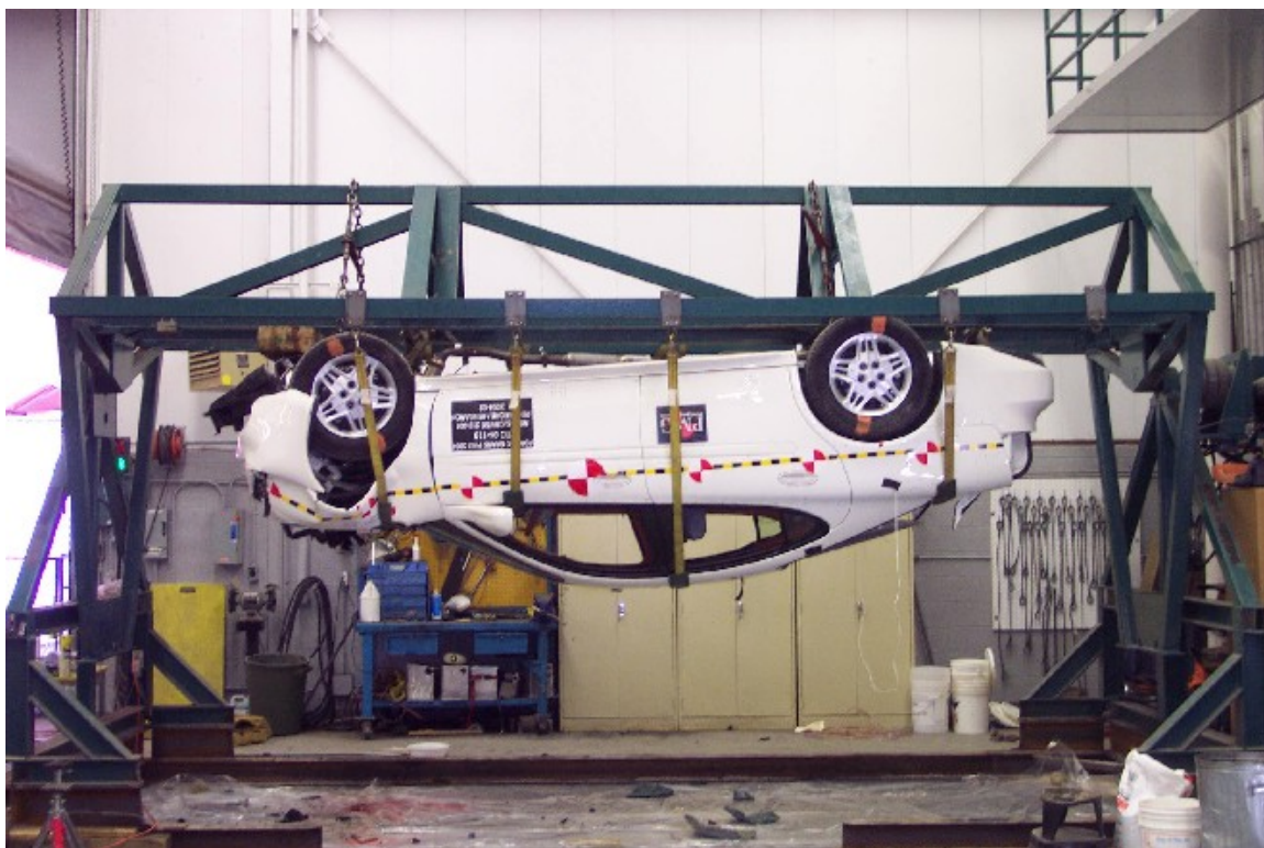
45. Vue du véhicule sur culbuteur à 180°. View of the vehicle on the roll over device at 180°.
