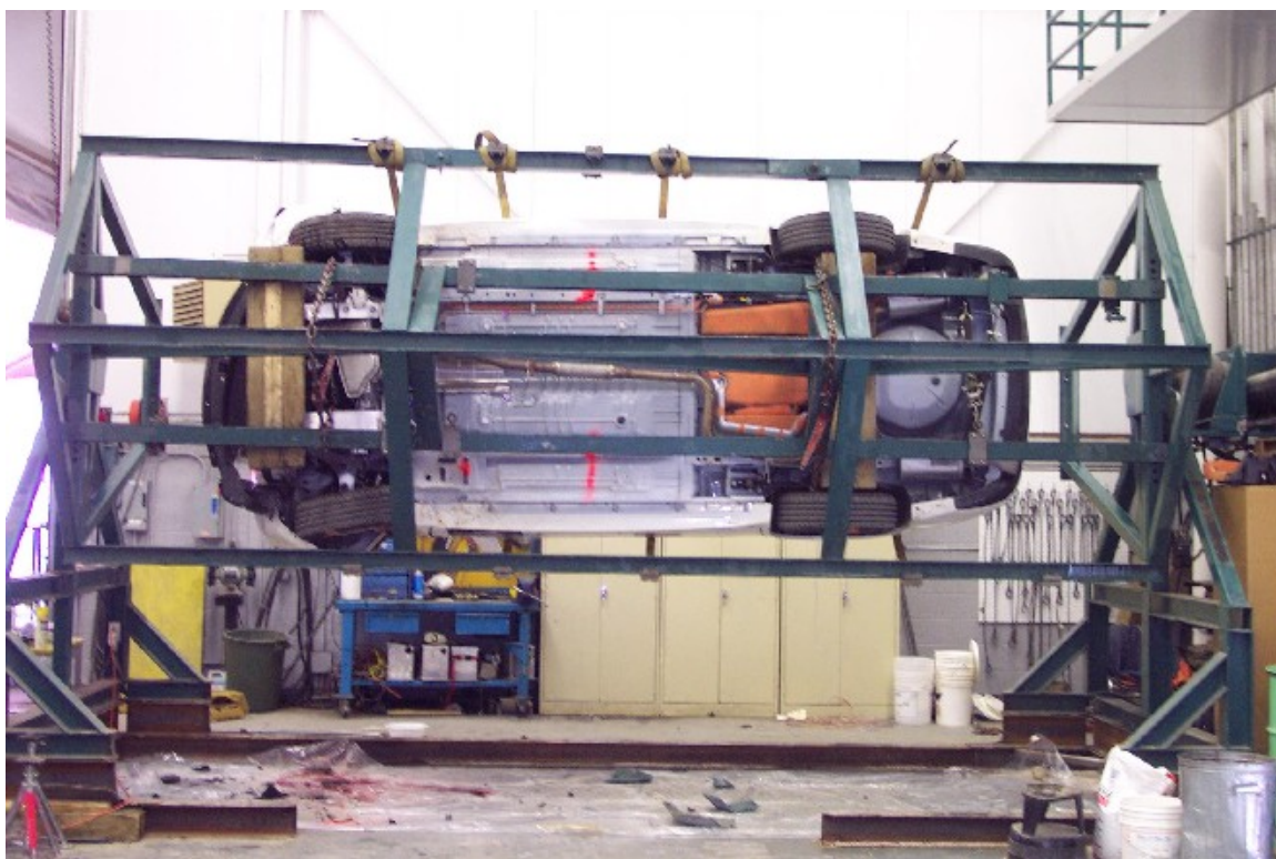
46. Vue du véhicule sur culbuteur à 270°. View of the vehicle on the roll over device at 270°.
