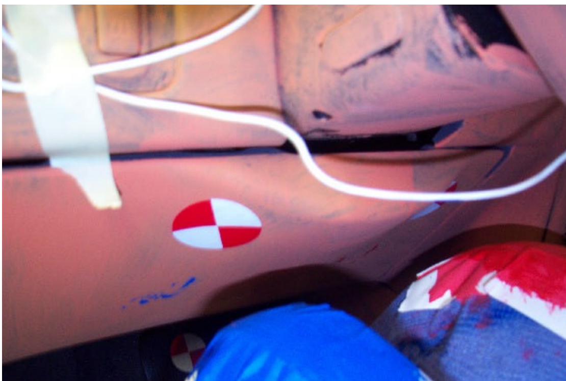
37. Point de contact des genoux du conducteur, après essai. Driver's knees contact point, post-test.
