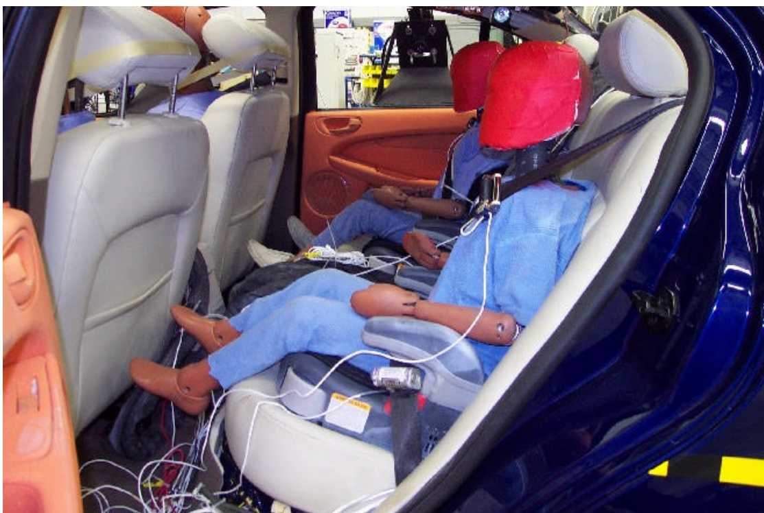
34. Position du passager arrière gauche, vue de gauche, avant essai. Rear left passenger's position, left side view, pre-test.
