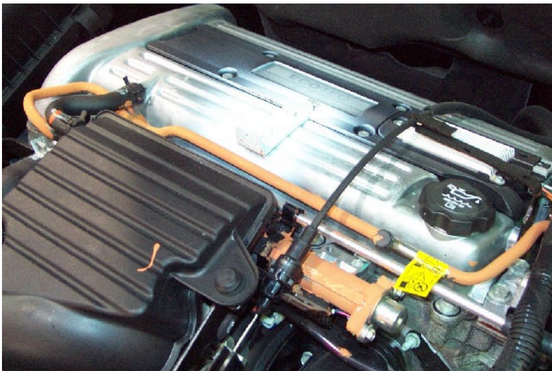
44. Lignes de carburant et vapeur dans le compartiment moteur. Filler and vapor lines in the engine compartment.
