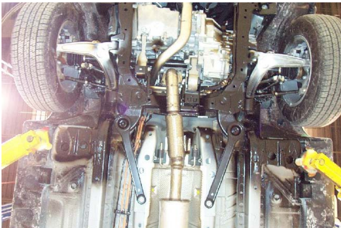
41. Vue du dessous du compartiment moteur, avant essai. Under view of the engine compartment , pre-test.
