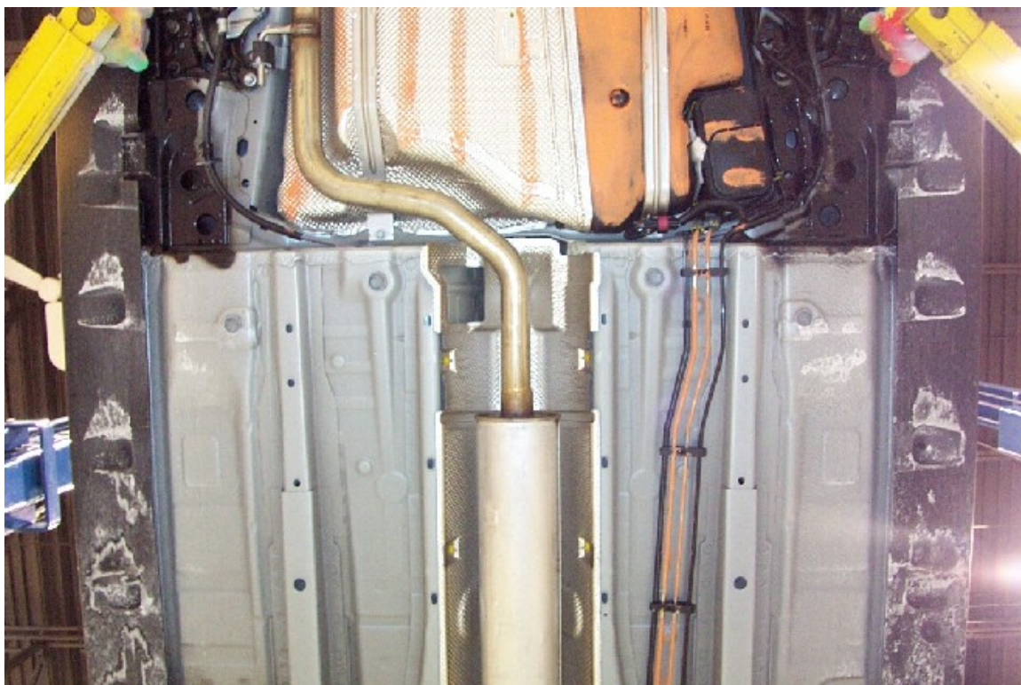
35. Ligne de carburant et vapeur. Fuel and vapor lines.
