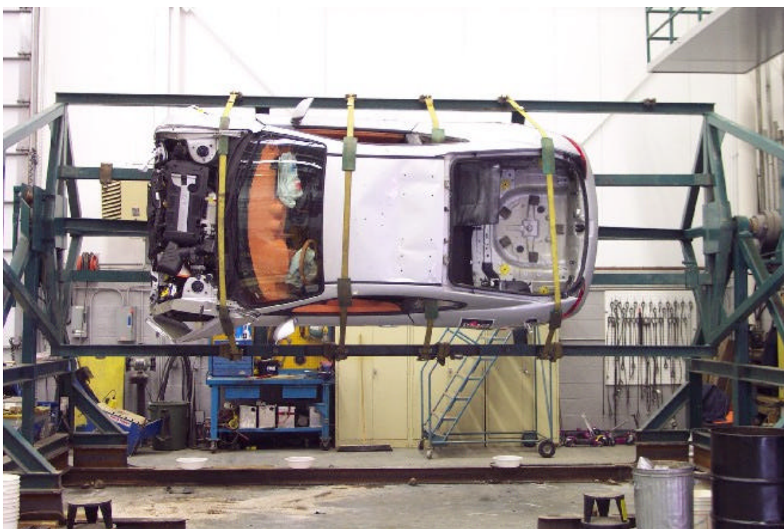
51. Vue du véhicule sur culbuteur à 90°. View of the vehicle on the roll over device at 90°.
