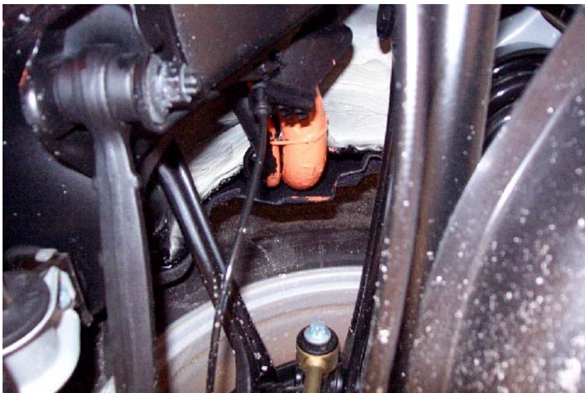
40. Tuyau de remplissage et vapeur. Filler and vapor pipe.
