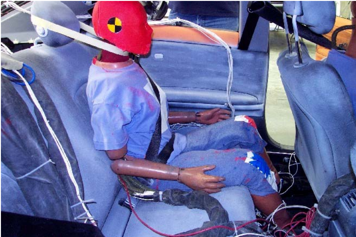
34. Position du passager arrière gauche, vue de droite, avant essai. Rear left passenger's position, right side view, pre-test.
