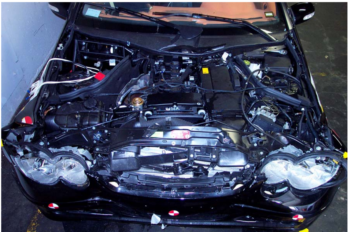
47. Vue du compartiment moteur du véhicule d'essai, après essai. Engine compartment view of the vehicle, post-test.
