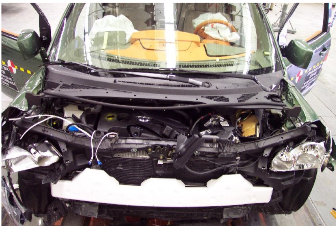
49. Vue du compartiment moteur du véhicule d'essai, après essai. Engine compartment view of the vehicle, post-test.
