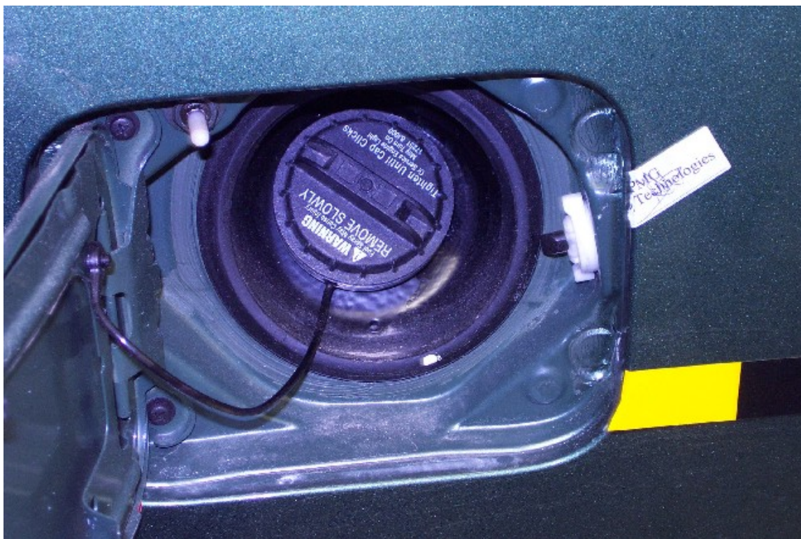
40. Bouchon de remplissage, avant essai. Filler cap, pre-test.
