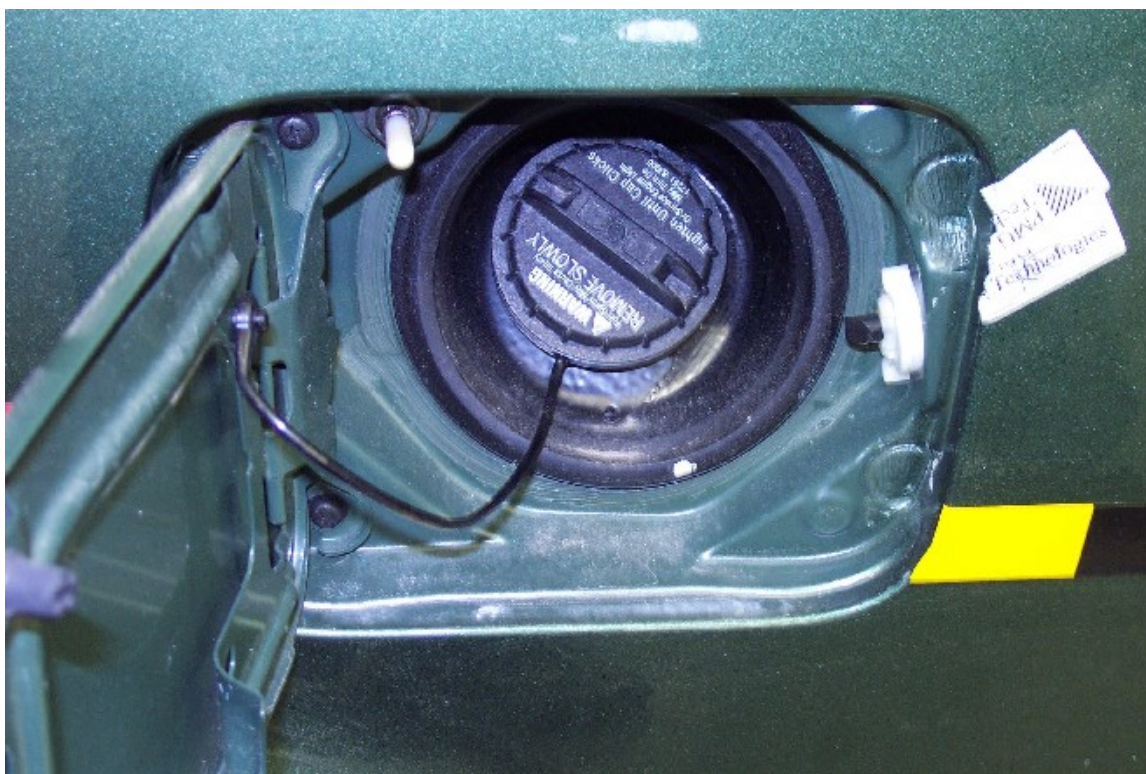
41. Bouchon de remplissage, après essai. Filler cap, post-test.
