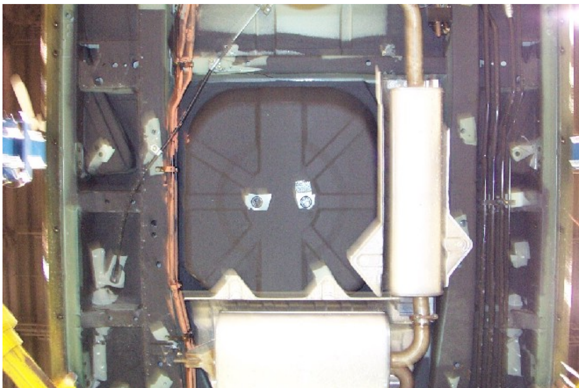
44. Ligne de carburant et vapeur. Fuel and vapor lines.
