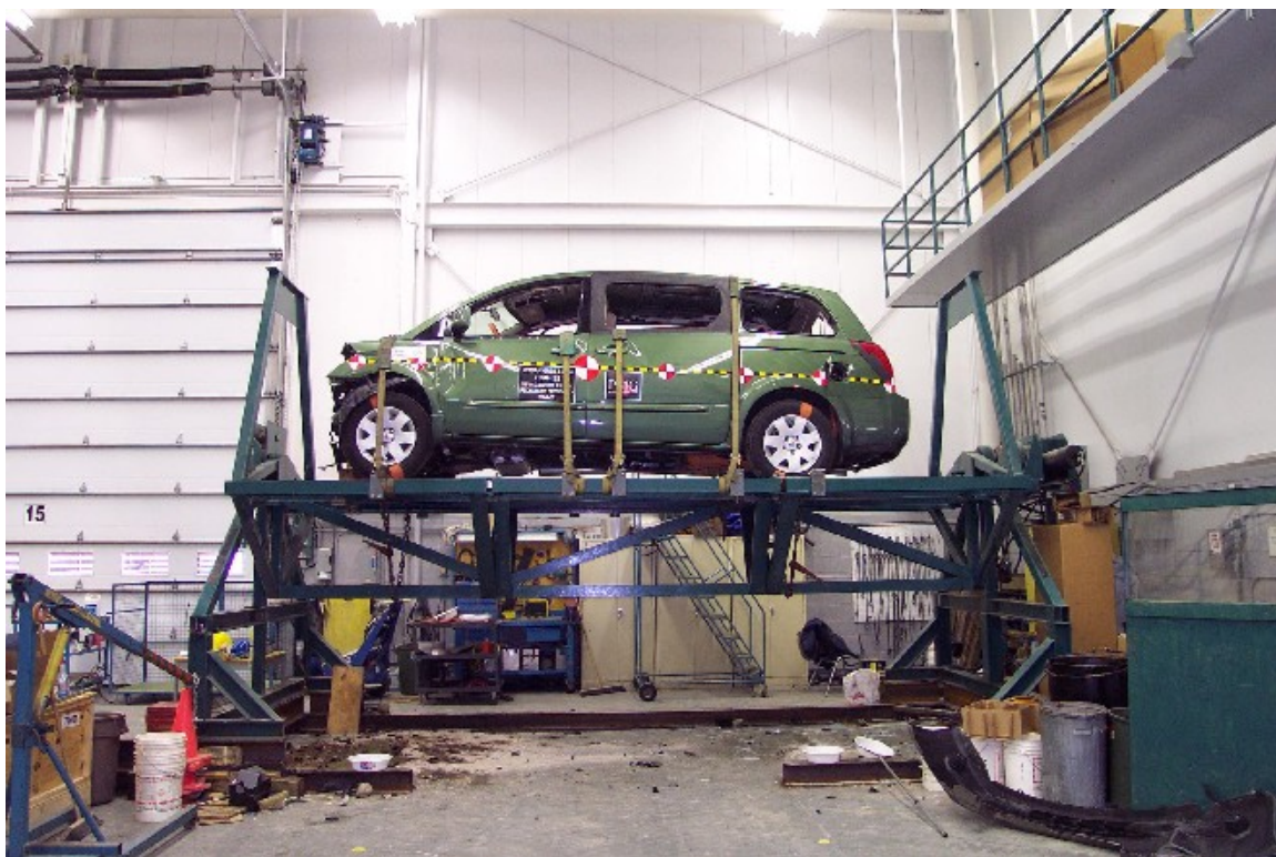
56. Vue du véhicule sur culbuteur à 360°. View of the vehicle on the roll over device at 360°.
