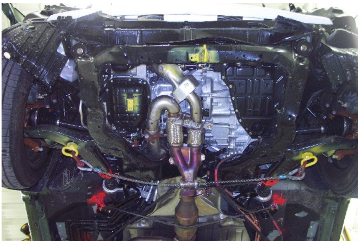
51. Vue du dessous du compartiment moteur, après essai. Under view of the engine compartment , post-test.
