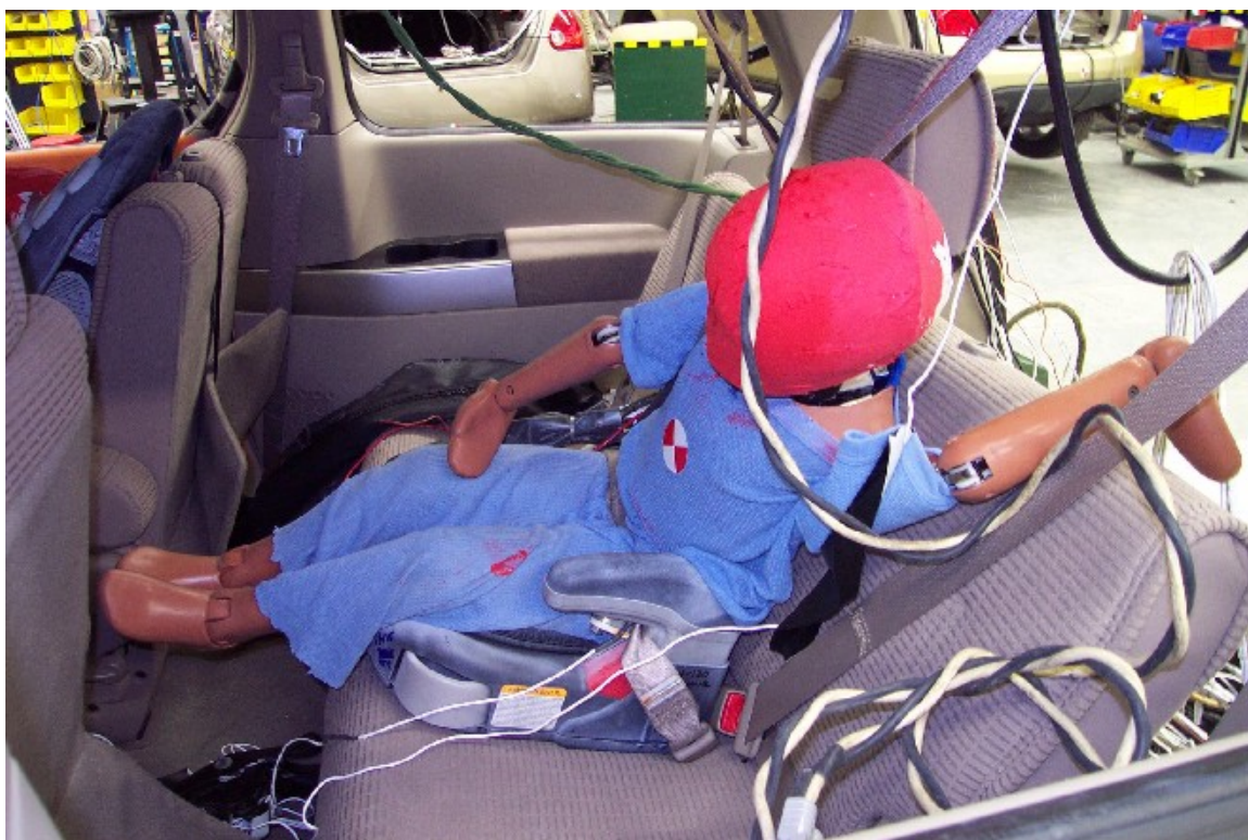
37. Position du passager arrière centre (3 e rangée), après essai. Rear center passenger's position (3 rd row), post-test.
