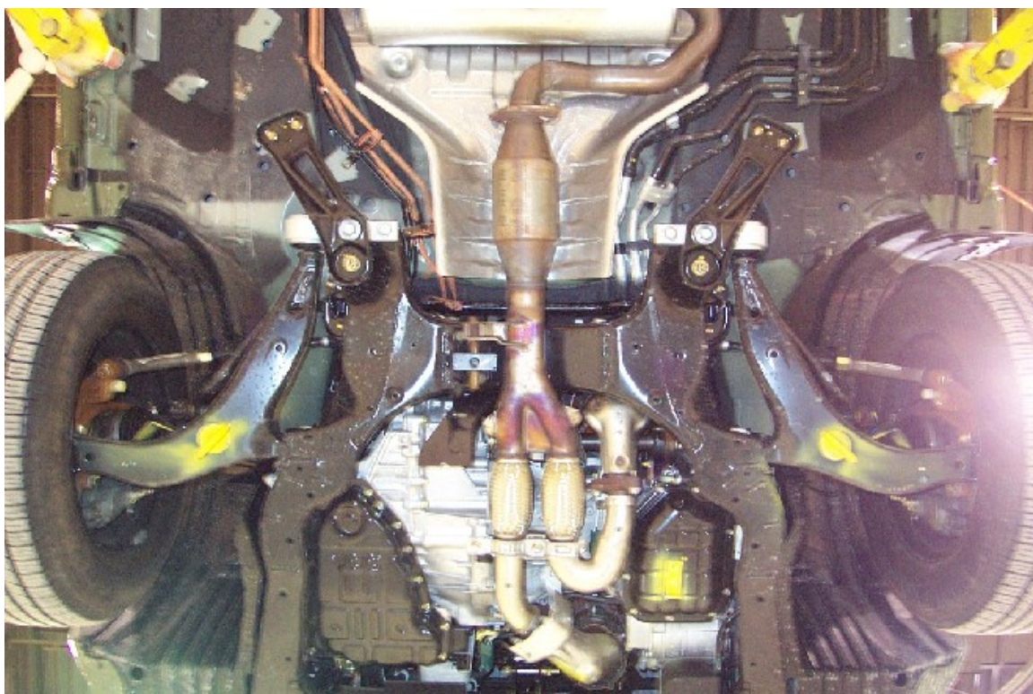
45. Lignes de carburant et vapeur. Fuel and vapor lines.
