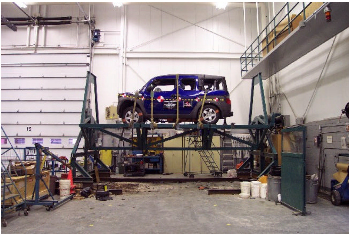
50. Vue du véhicule sur culbuteur avant l'essai de capotage statique. View of the vehicle on the roll over device before testing.
