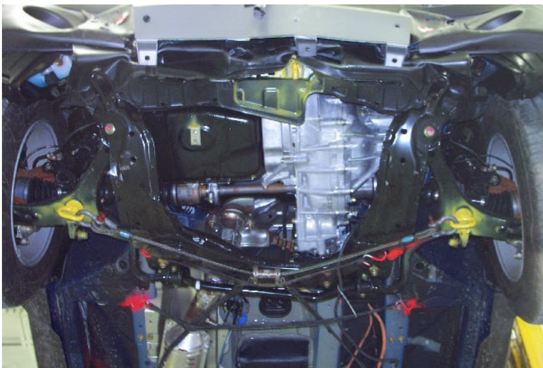
49. Vue du dessous du compartiment moteur, après essai. Under view of the engine compartment , post-test.
