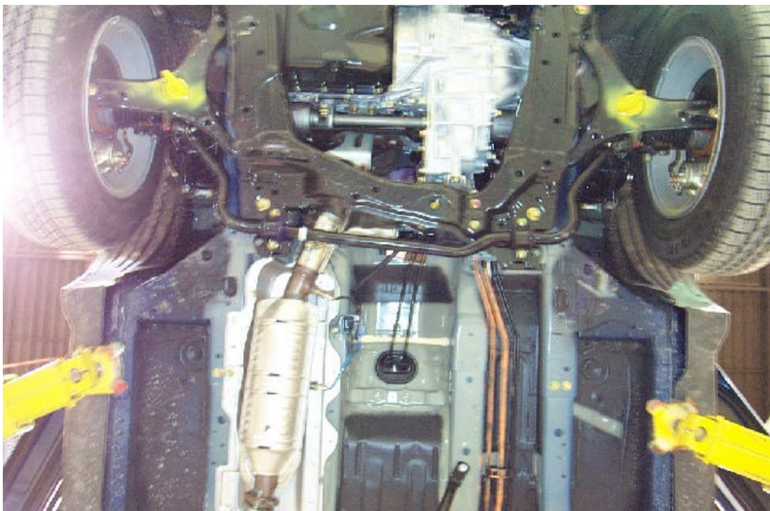
48. Vue du dessous du compartiment moteur, avant essai Under view of the engine compartment , pre-test.
