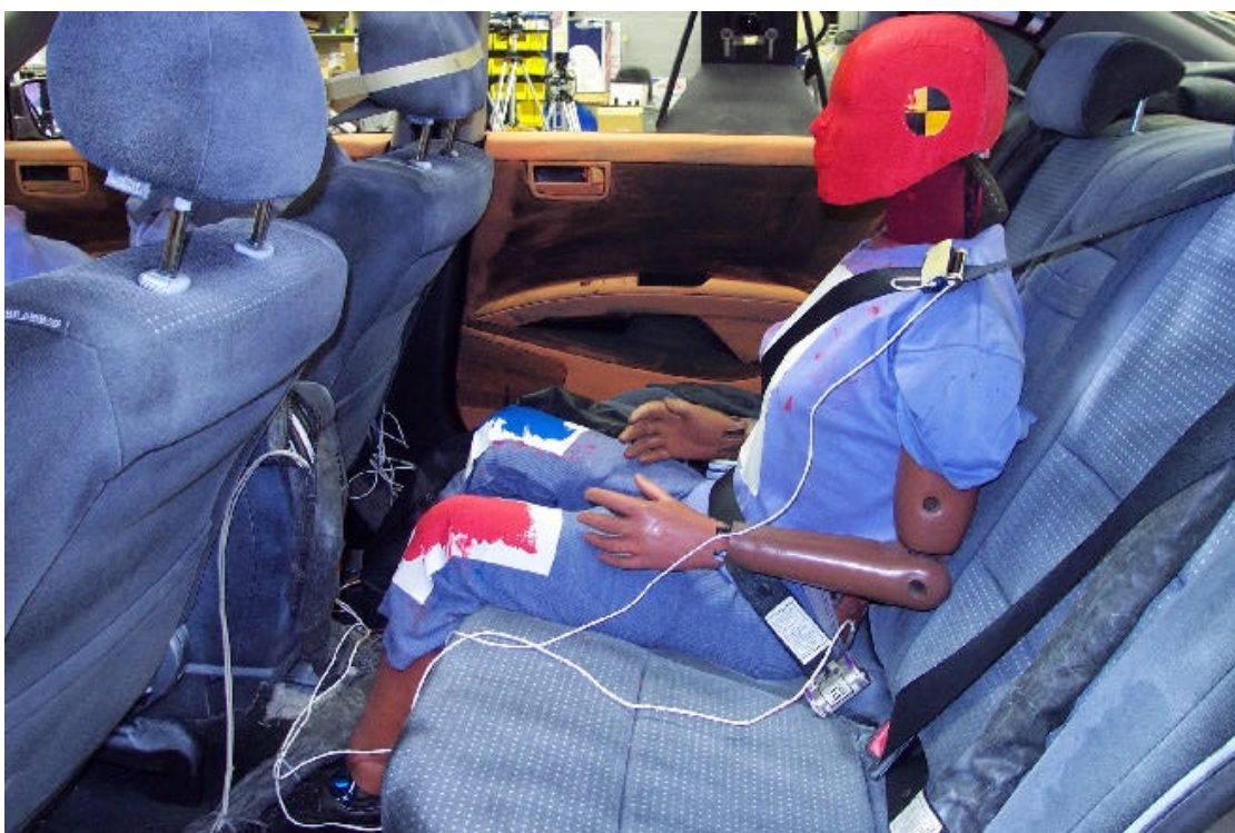
32. Position du passager arrière centre, vue de gauche, avant essai. Rear centre passenger's position, left side view, pre-test.
