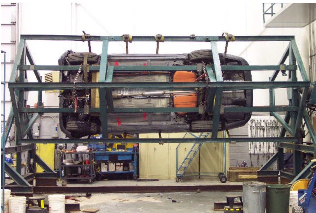
53. Vue du véhicule sur culbuteur à 270°. View of the vehicle on the roll over device at 270°.
