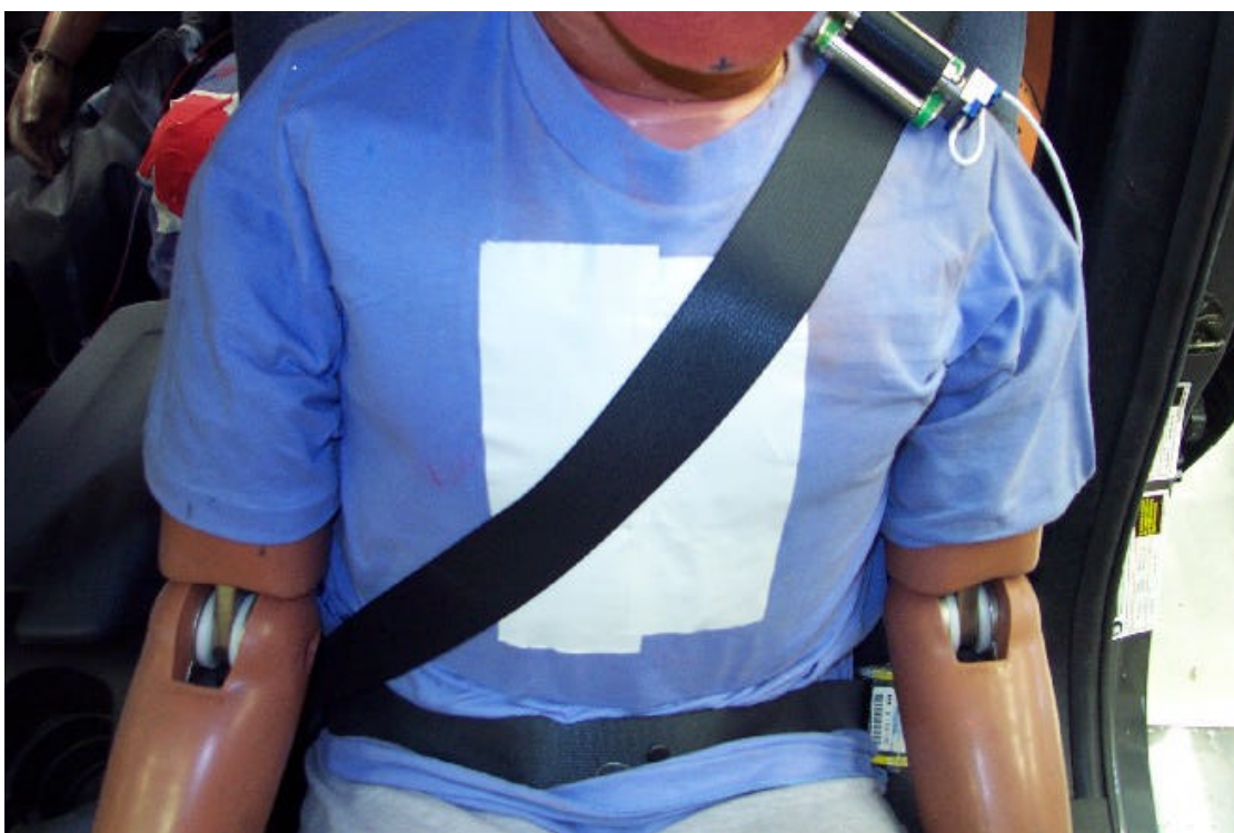
26. Contact du volant sur l'abdomen du conducteur, après essai. Steering wheel's contact point with driver's abdomen.
