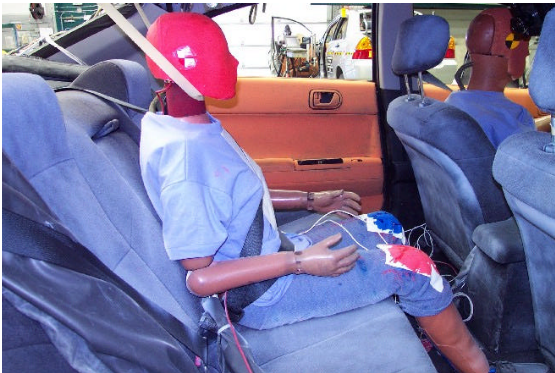
34. Position du passager arrière centre, vue de droite, avant essai. Rear center passenger's position, right side view, pre-test.
