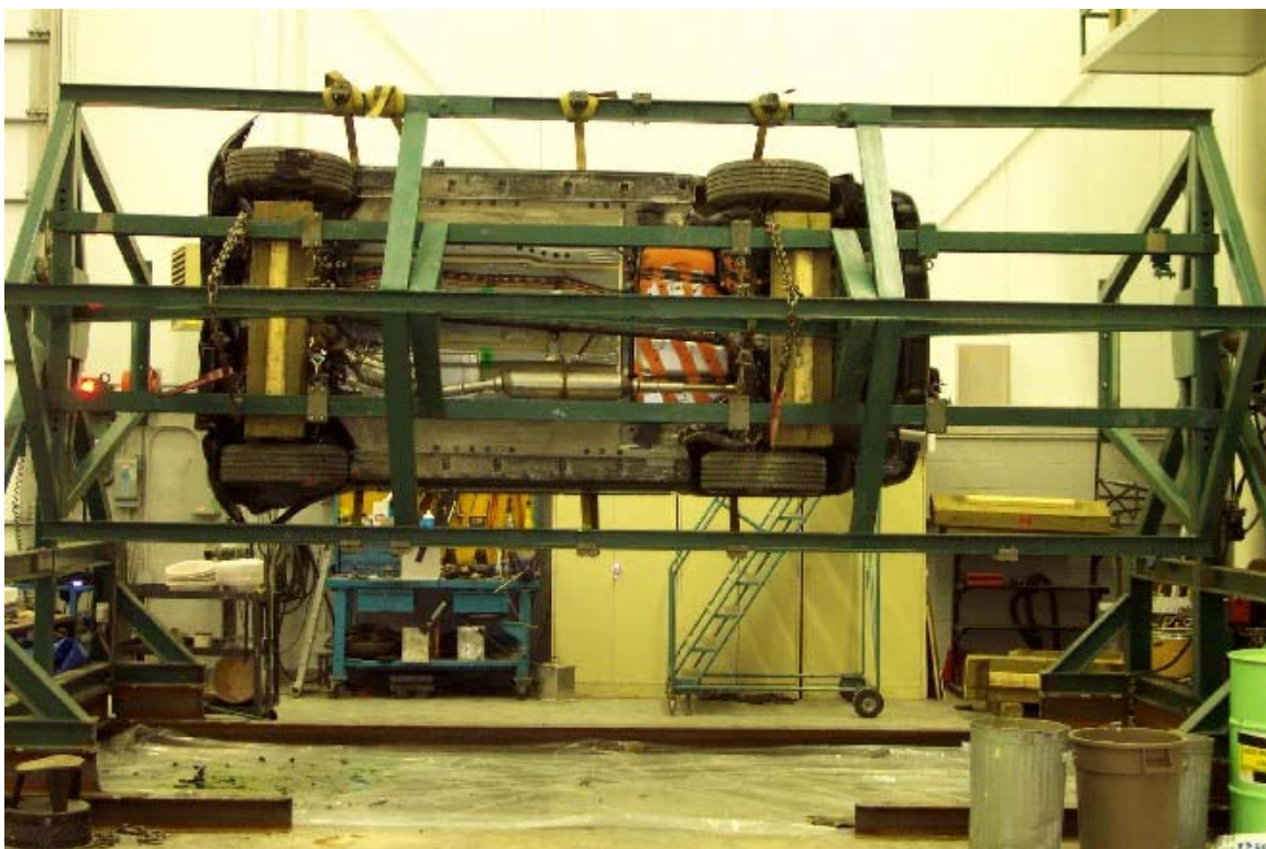
44. Vue du véhicule sur culbuteur à 270°. View of the vehicle on the roll over device at 270°.
