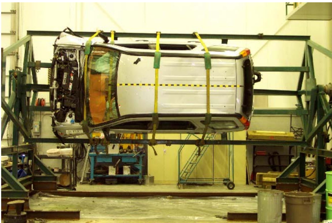
42. Vue du véhicule sur culbuteur à 90°. View of the vehicle on the roll over device at 90°.
