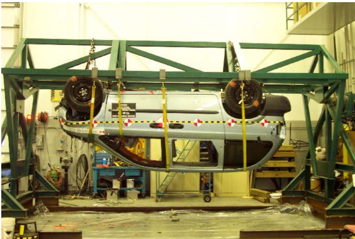
51. Vue du véhicule sur culbuteur à 180°. View of the vehicle on the roll over device at 180°.
