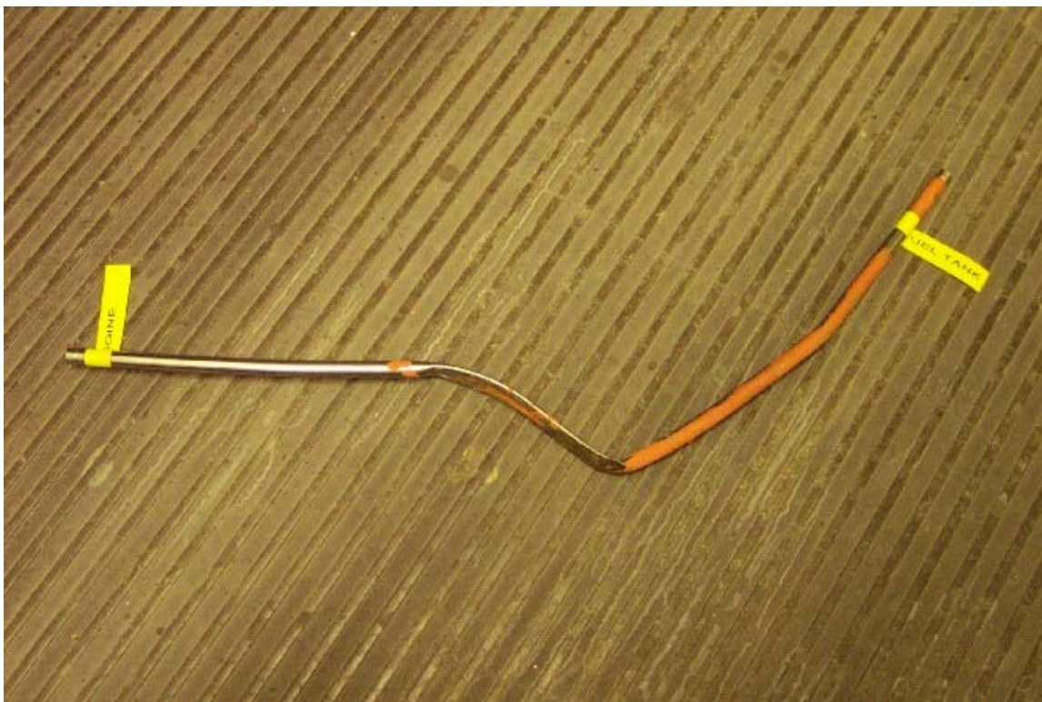
54. Vue de la conduite d'alimentation de carburant, après essai. View of the fuel supply line, post-test.
