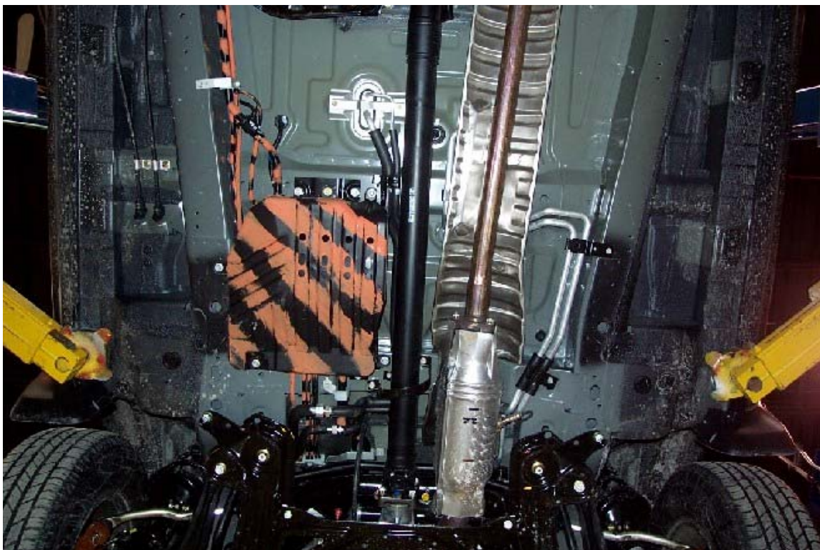
38. Ligne de carburant et vapeur. Fuel and vapor lines.
