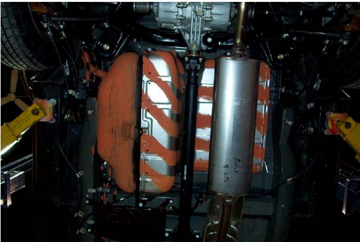
37. Réservoir de carburant. Fuel tank.
