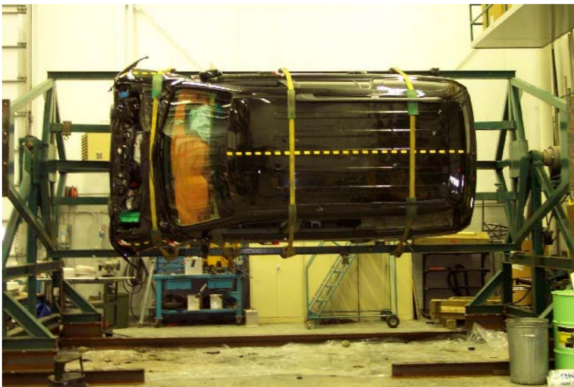
47. Vue du véhicule sur culbuteur à 90°. View of the vehicle on the roll over device at 90°.
