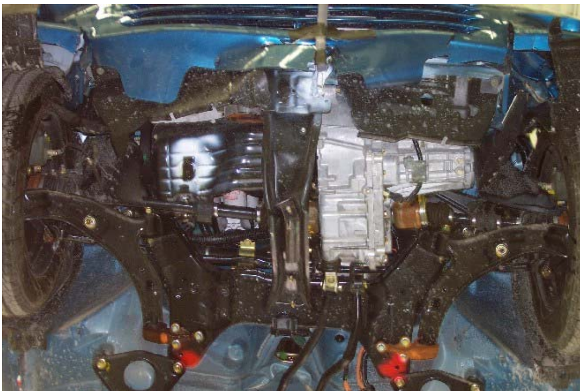
45. Vue du dessous du compartiment moteur, après essai. Under view of the engine compartment , post-test.
