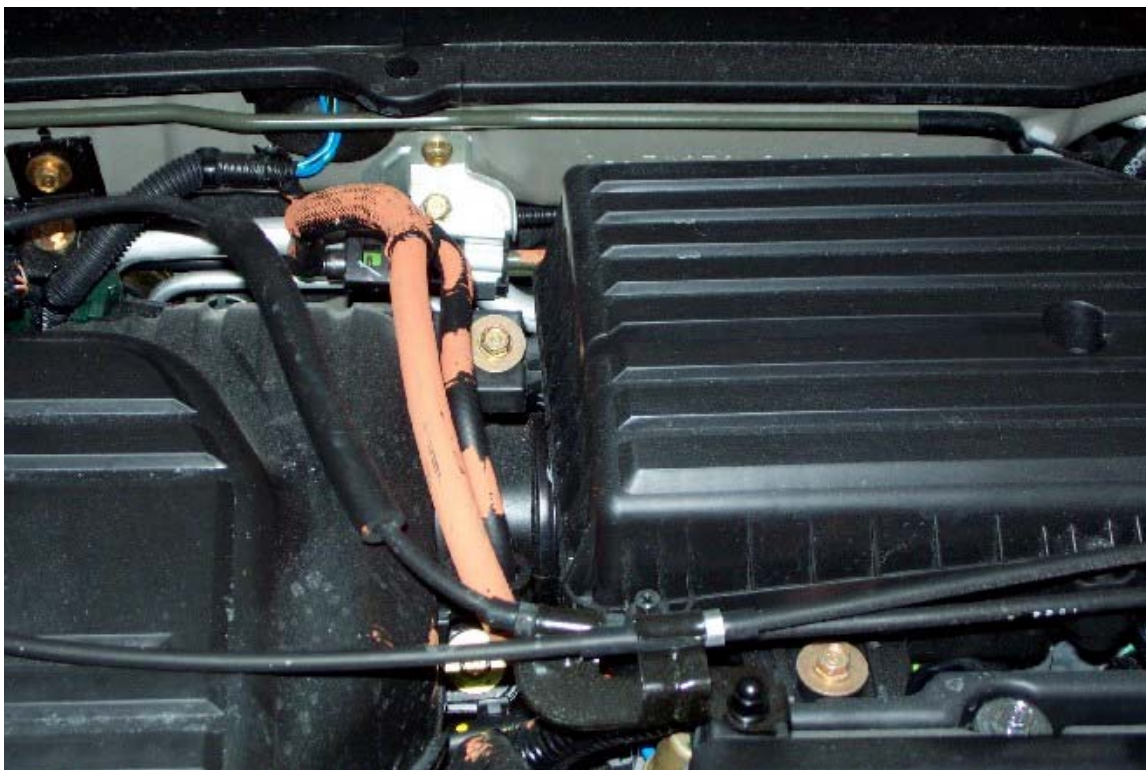
37. Lignes de carburant et vapeur dans le compartiment moteur. Filler and vapor lines in the engine compartment.
