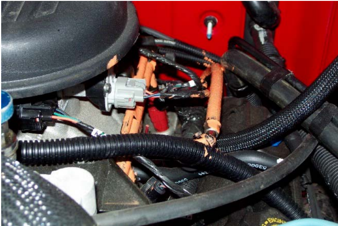
33. Lignes de carburant et vapeur dans le compartiment moteur. Filler and vapor lines in the engine compartment.
