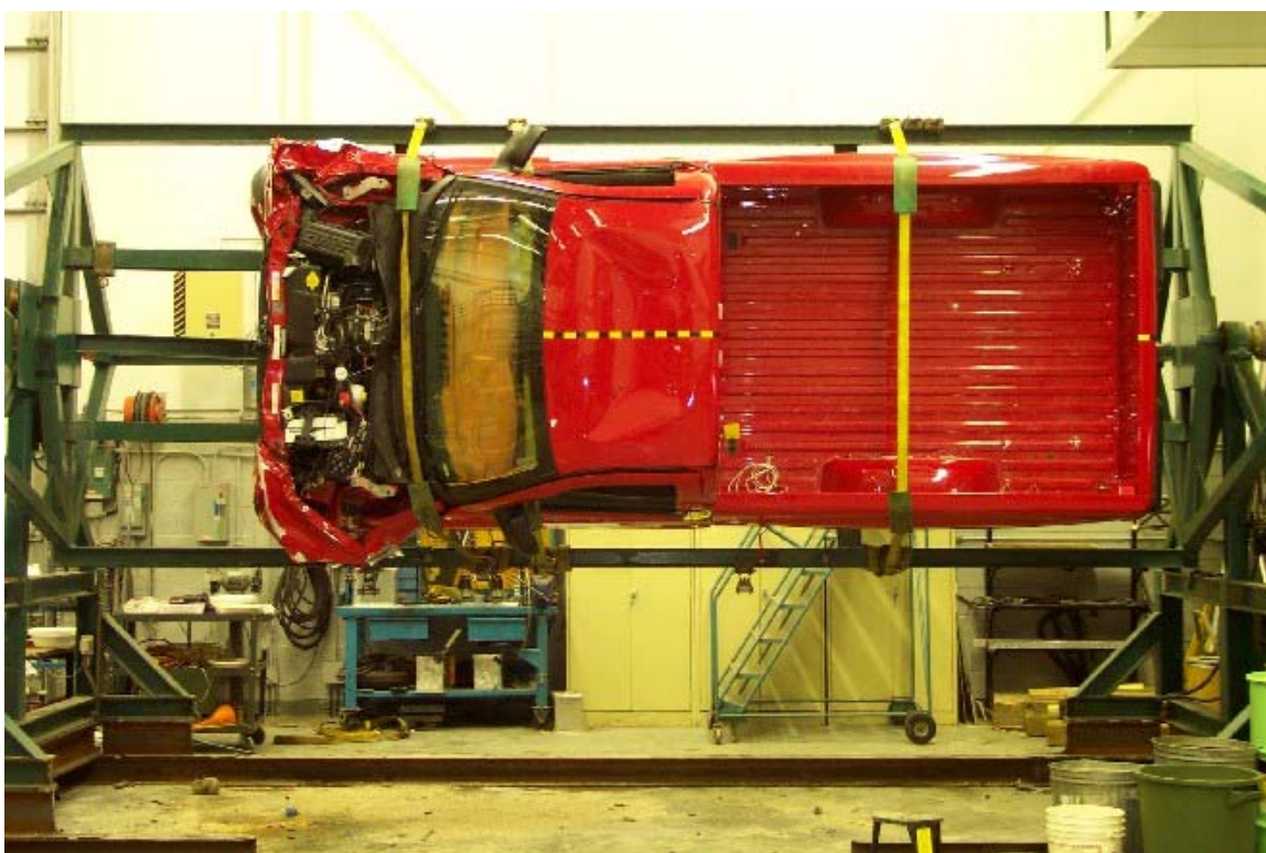
40. Vue du véhicule sur culbuteur à 90°. View of the vehicle on the roll over device at 90°.
