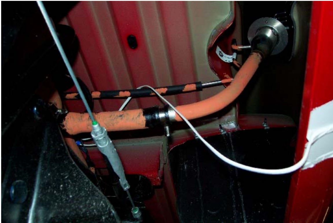
29. Tuyau de remplissage et vapeur. Filler and vapor pipe.
