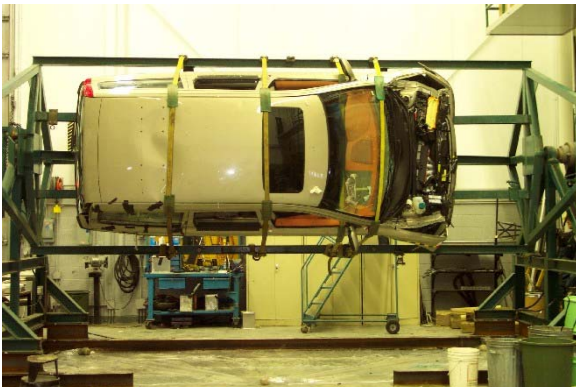
44. Vue du véhicule sur culbuteur à 90°. View of the vehicle on the roll over device at 90°.
