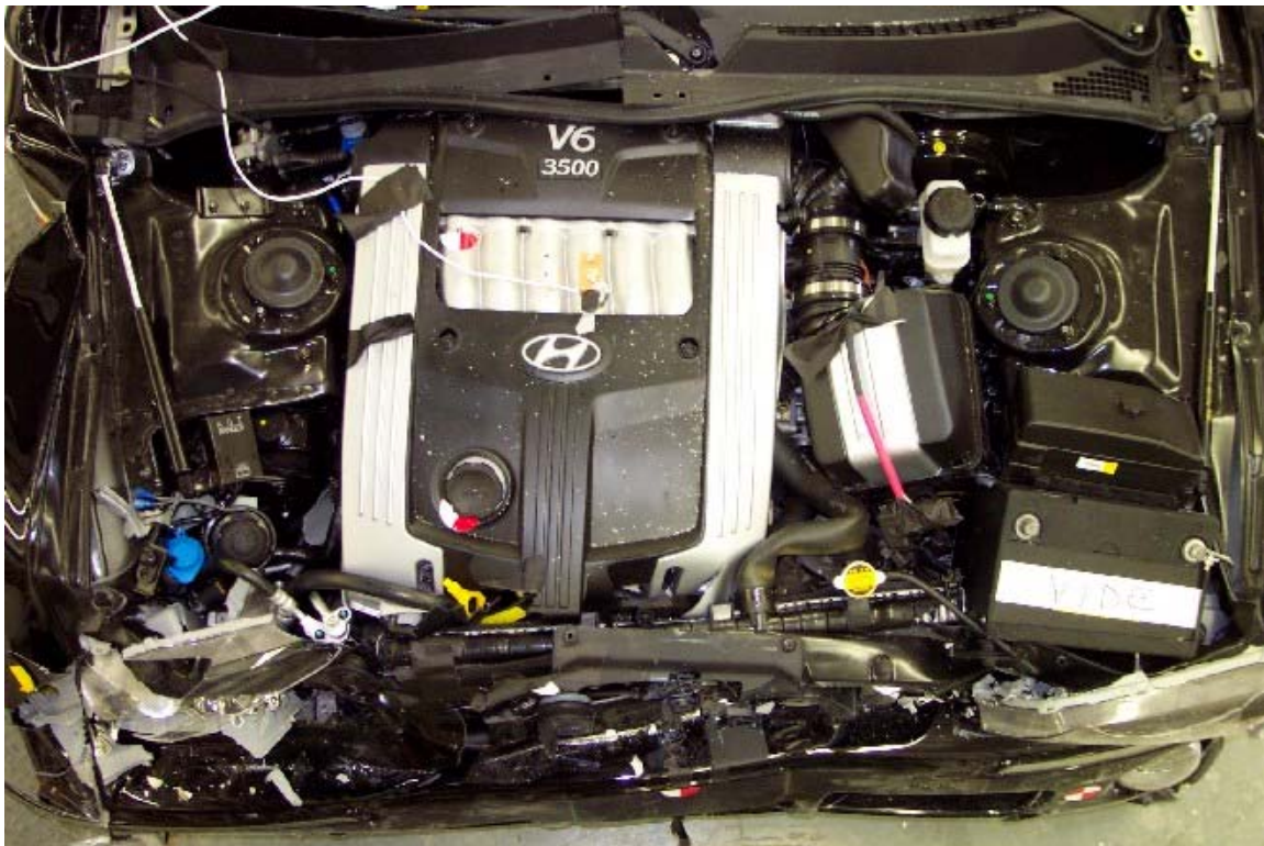
43. Vue du compartiment moteur du véhicule d'essai, après essai. Engine compartment view of the vehicle, post-test.
