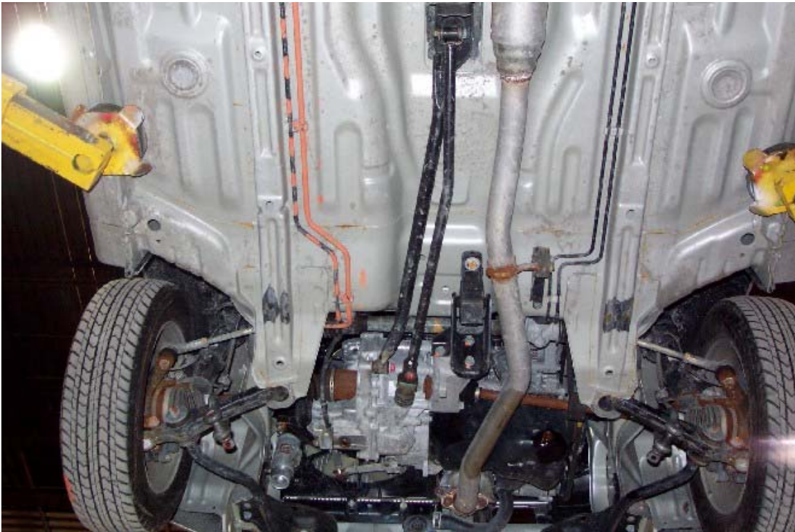
37. Ligne de carburant et vapeur. Fuel and vapor lines.
