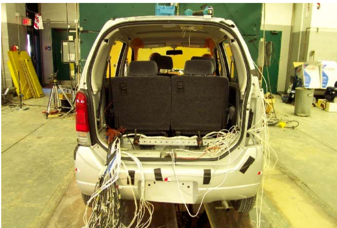
7. Vue arrière du véhicule d'essai, après essai. Rear view of the test vehicle, post-test.
