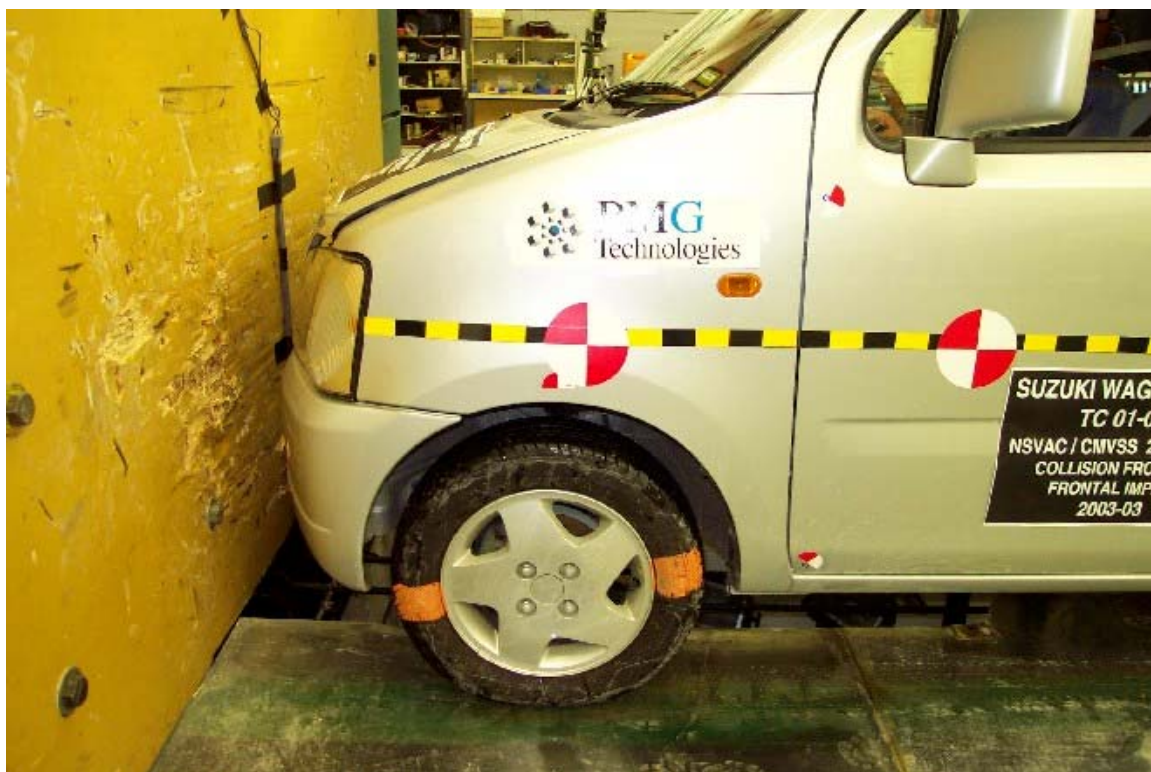
16. Vue côté gauche de l'avant du véhicule d'essai, avant essai. Left side view of front of test vehicle, pre-test.
