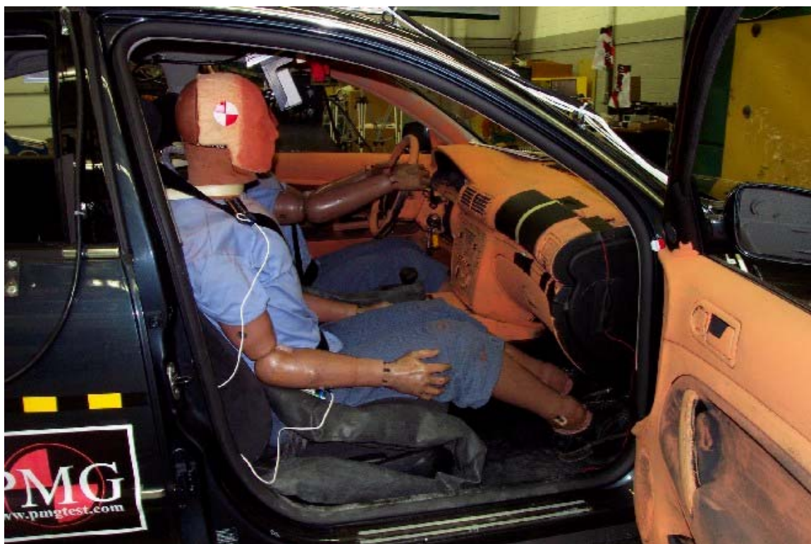
27. Position du passager, avant essai. Passenger's position, pre-test.
