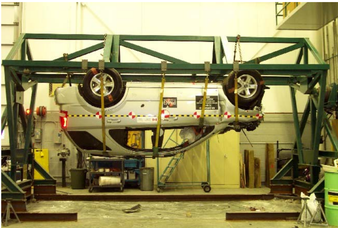
48. Vue du véhicule sur culbuteur à 180°. View of the vehicle on the roll over device at 180°.
