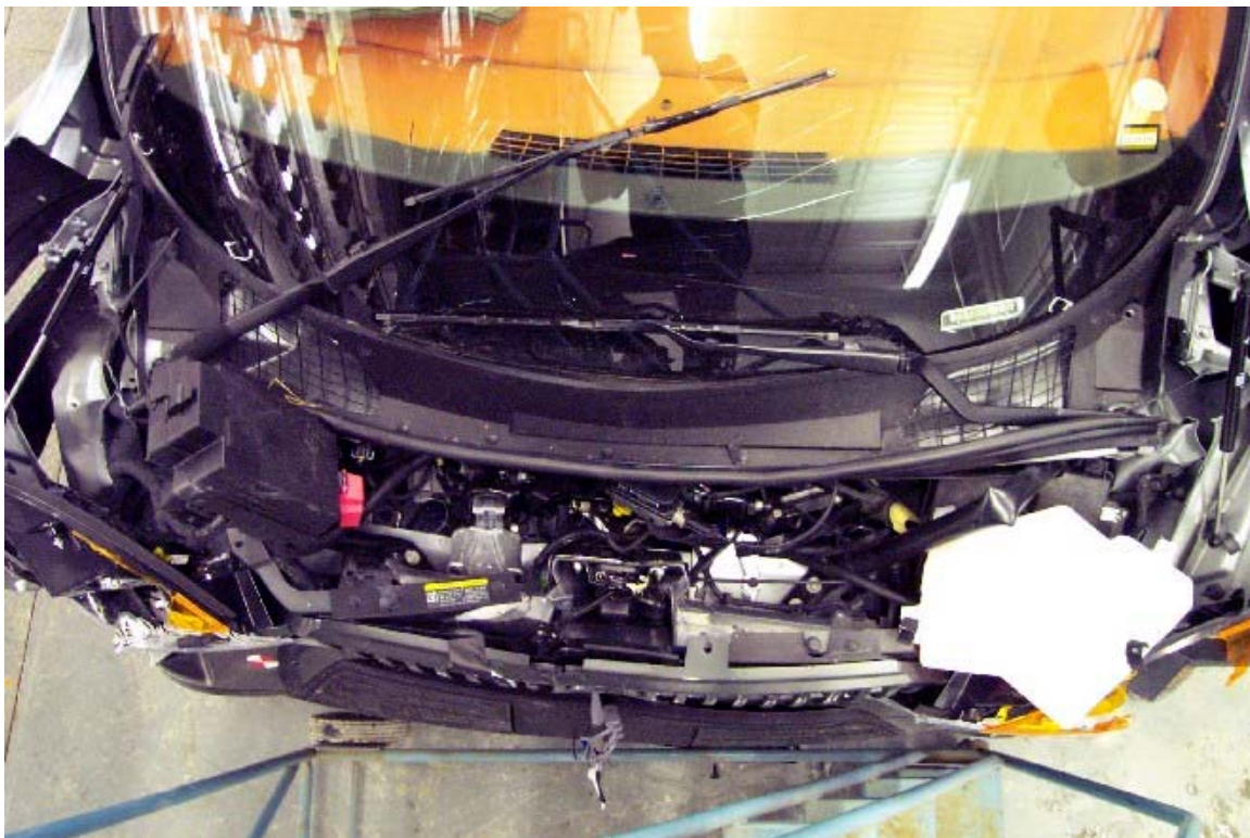
40. Vue du compartiment moteur du véhicule d'essai, après essai. Engine compartment view of the vehicle, post-test.
