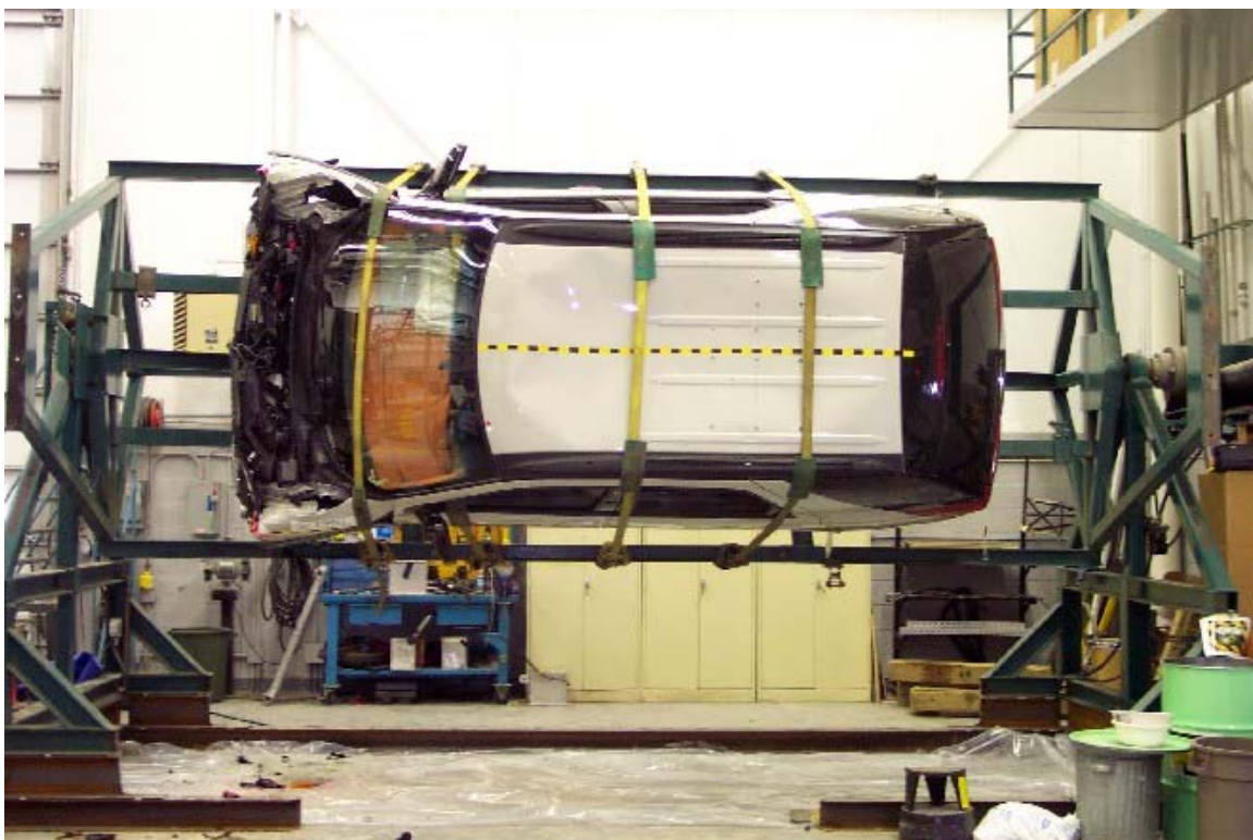
49. Vue du véhicule sur culbuteur à 90°. View of the vehicle on the roll over device at 90°.
