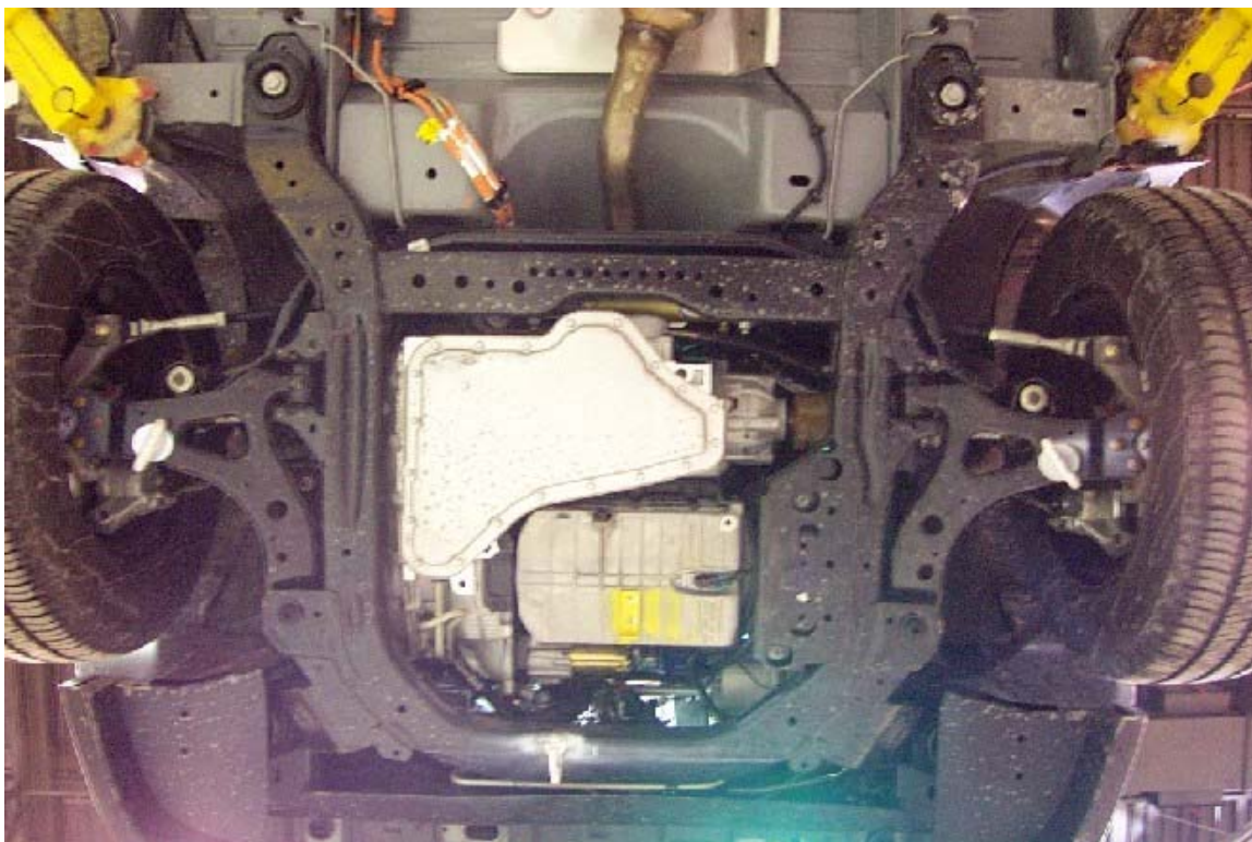
46. Vue du dessous du compartiment moteur, avant essai. Under view of the engine compartment , pre-test.
