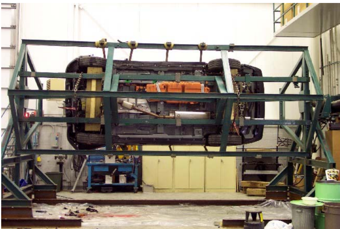
51. Vue du véhicule sur culbuteur à 270°. View of the vehicle on the roll over device at 270°.
