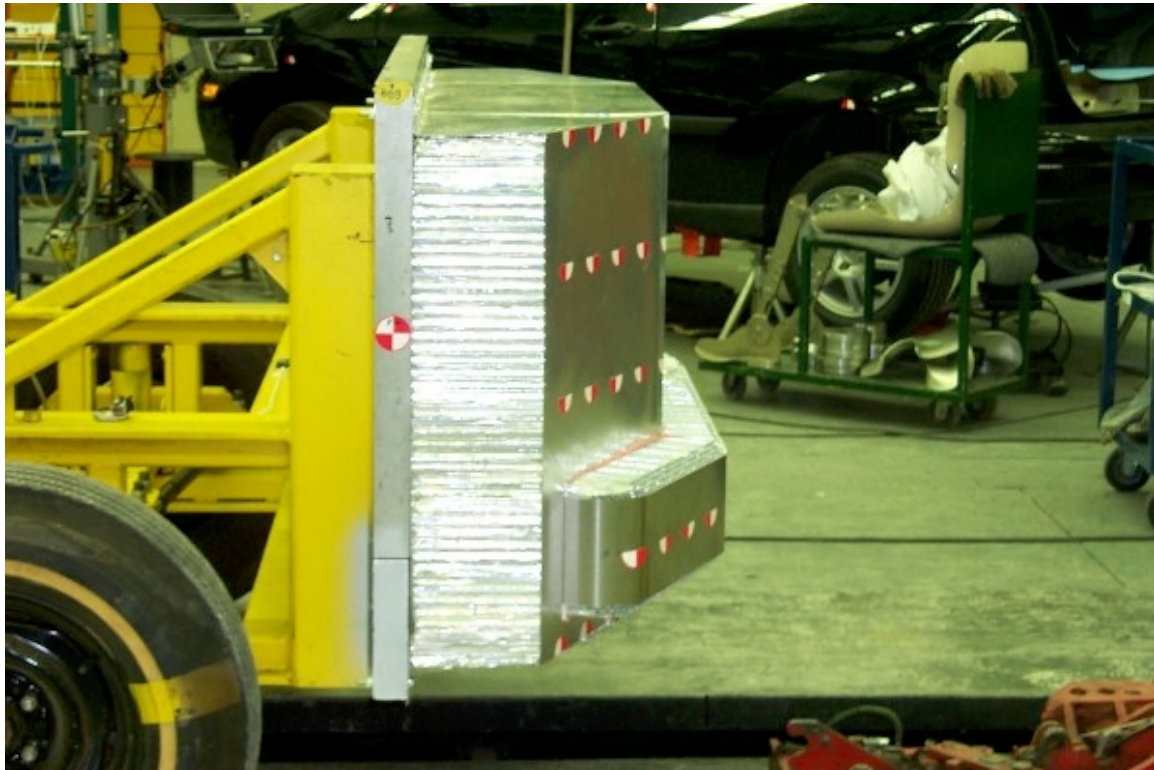
21. Vue du côté droit de la face déformable, avant essai. Right side view of the deformable face, pre-test.
