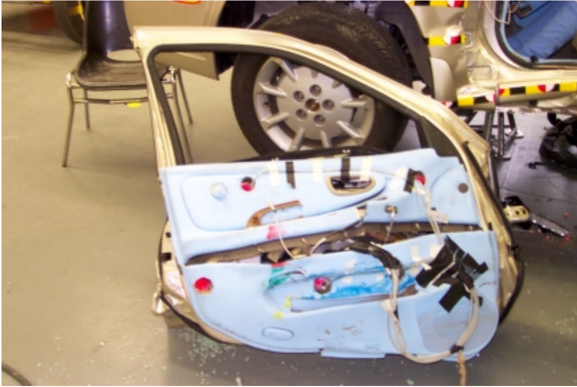
50. Points de contact sur l'intérieur de la portière avant gauche, après essai. Contact points on the inside of the left front door trim, post-test .
