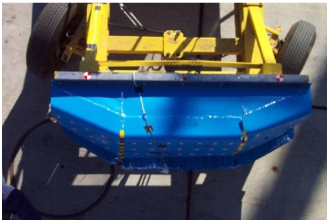
24. Vue de plan de la face déformable, après essai. Overview of the deformable face, post-test.
