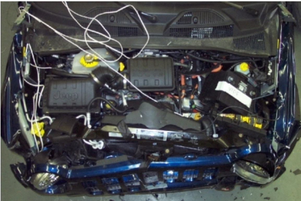
36. Vue du compartiment moteur du véhicule d'essai, après essai. Engine compartment view of the vehicle, post-test.
