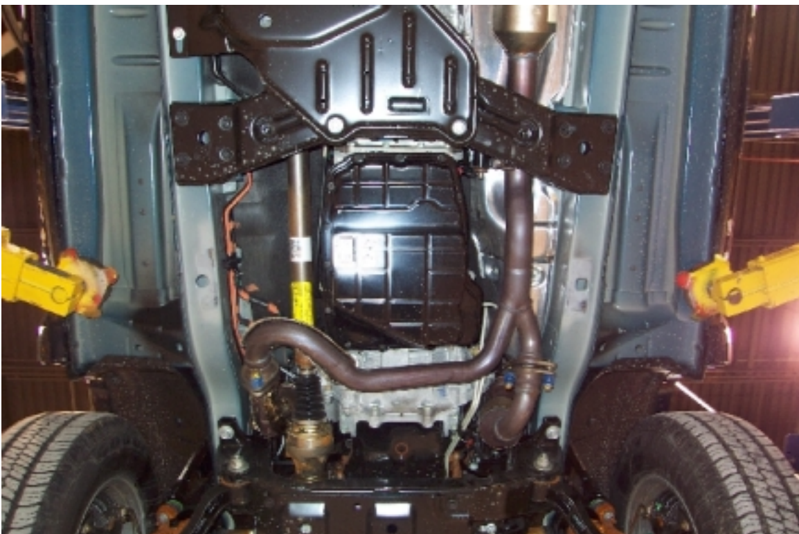
32. Lignes de carburant et vapeur. Fuel and vapor lines.
