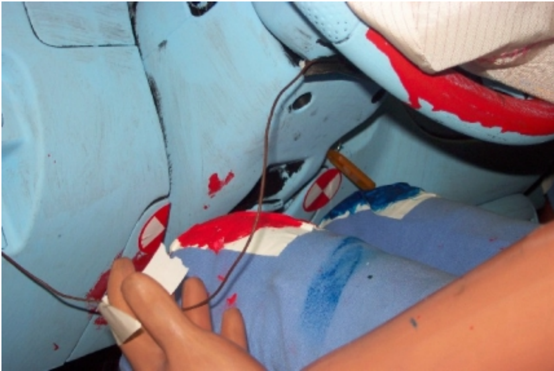
35. Point de contact des genoux du conducteur, après essai. Driver's knee contact points, post-test.
