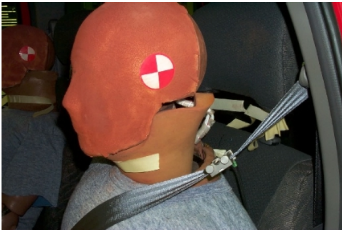
32. Point de contact de tête du conducteur, après essai. Driver's head contact point, post-test.
