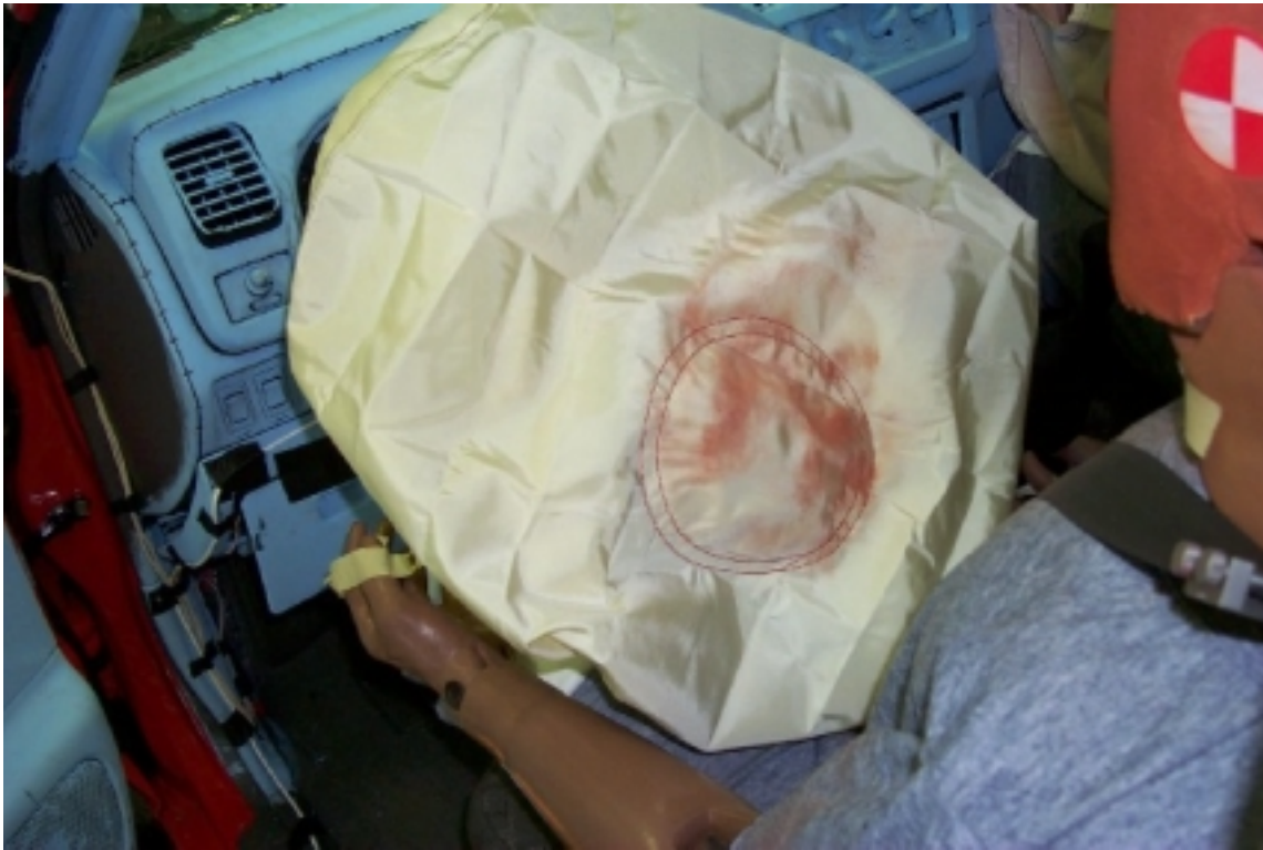
31. Point de contact de tête du conducteur, après essai. Driver's head contact point, post-test.
