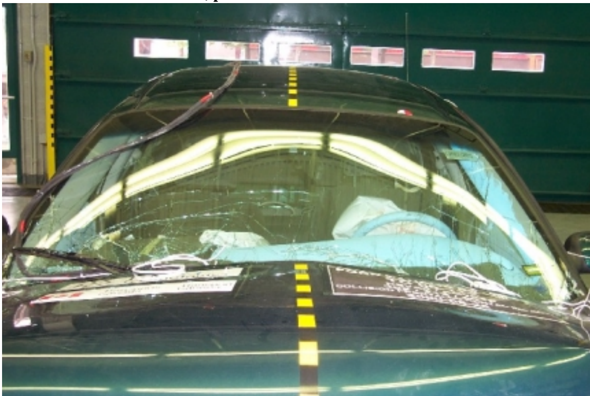
26. Pare-brise, après essai. Windshield, post-test.
